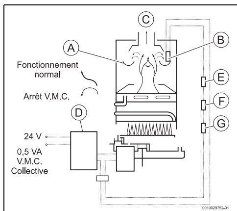
Fig. 27 Schéma de principe V.M.C.
