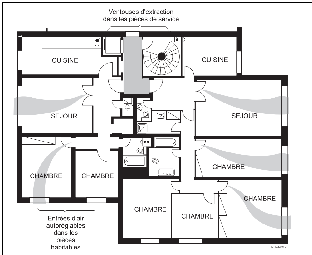
Fig. 26 Schéma de ventilation mécanique contrôlée de locaux d'habitation
