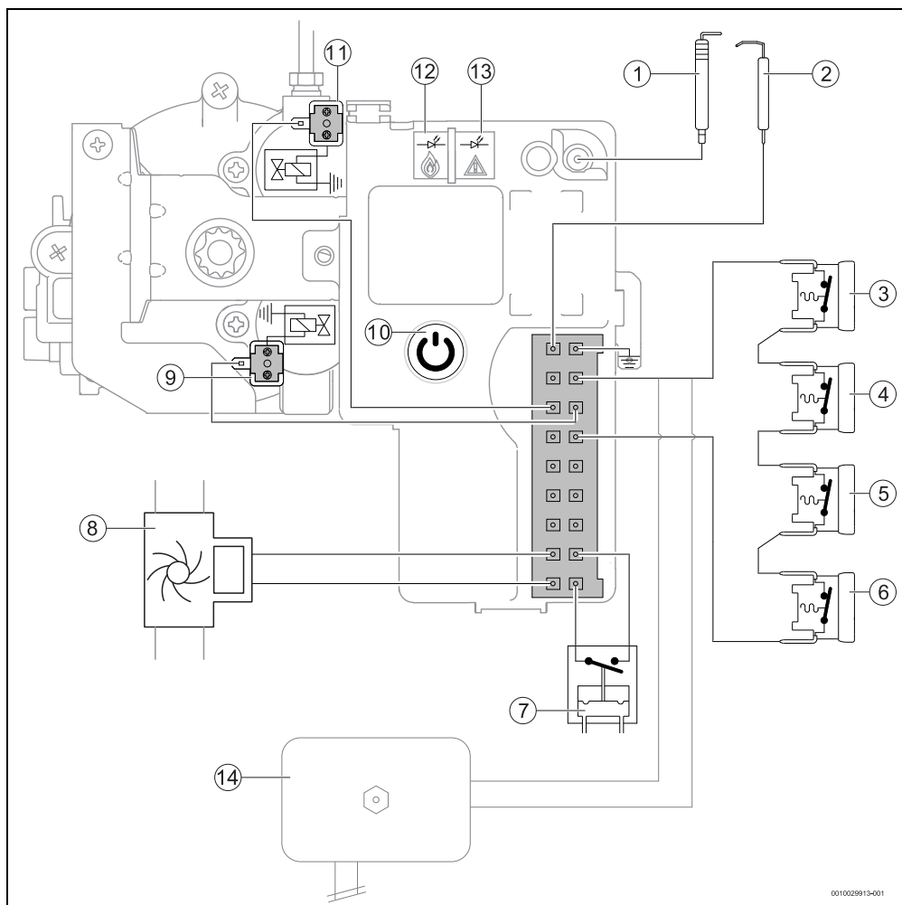
Fig. 29 Schéma de connexion
