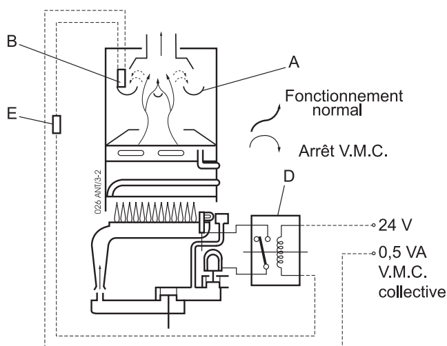
Schéma de principe
