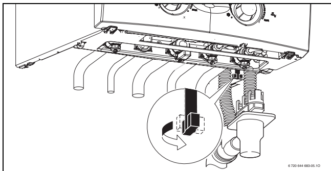
Fig. 5 Robinet de remplissage
