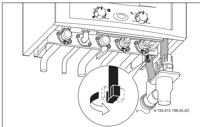
Fig. 6 Robinet de remplissage (appareils GVAC)
