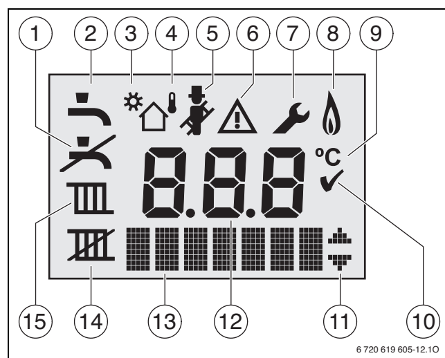
Fig. 2 Symboles d'affichage
