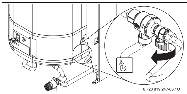
Fig. 4 Dispositif de remplissage du ballon BIL50M
