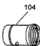
Récupérateur de condensats Ø 80/125 CFFVF0007 Ø 100/150 CFFVF0036
