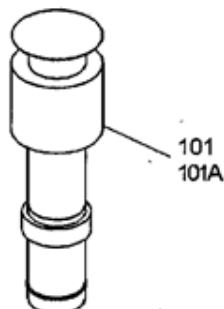
Terminal vertical 101 Ø 80/125 CFFVF0013 brique Ø 100/150 CFF0037 brique 101A Ø 80/125 CFFVF0015 noir Ø 100/150 CFFVF0038
