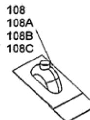
108 Solin tuile 10° à 30° base plomb Ø 80/125 CFFVF0011 Ø 100/150 CFFVF0045 108A Solin tuile 30° à 45° base plomb Ø 80/125 CFFVF0012 Ø 100/150 CFFVF0046 108B Solin ardoise 30° à 45° Ø 80/125 CFFVF0014 Ø 100/150 CFFVF0048 108C Solin toit plat Ø 80/125 CFFVF0050 Ø 100/150 CFFVF0047
