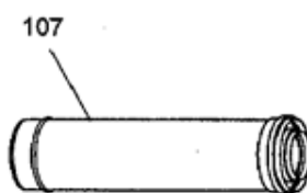
Rallonge télescopique Ø 80/125 CFFVF0010 Ø 100/150 CFFVF0041
