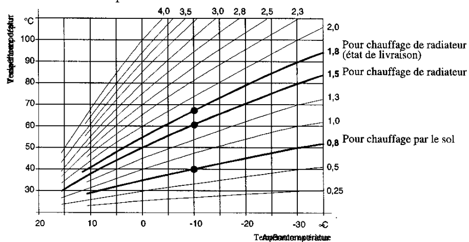
Fig. 3 Diagramme des courbes caractéristiques de chauffe
