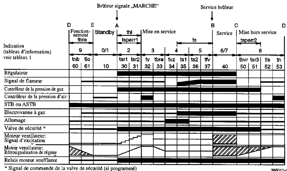
Fig. 11 Déroulement du programme Centrale de commande et de régulation LGM 11.44 A 2590
