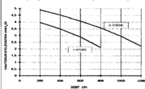
23 FF - pompe surdimensionnée (sur demande)
