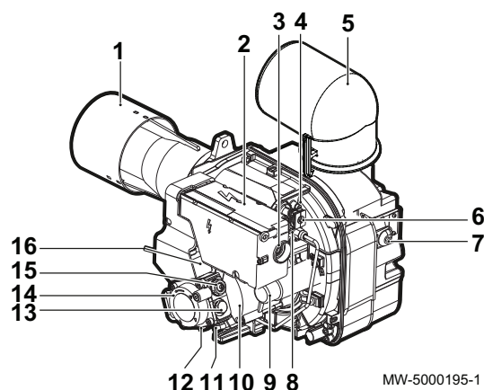
Fig.3 Principaux composants
