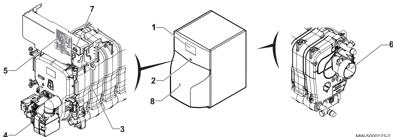
Fig.2 Principaux composants
