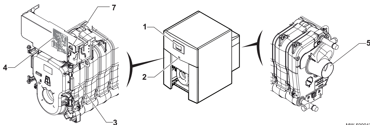
Fig.2 Principaux composants
