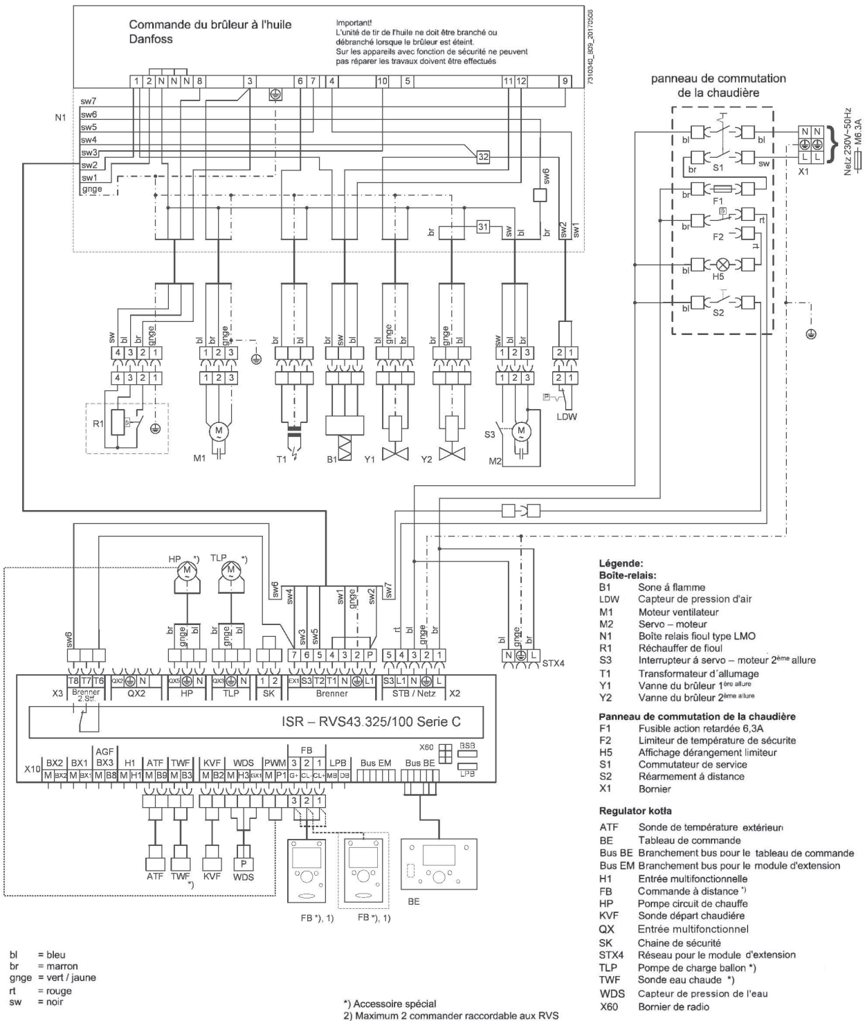
Fig.4 Schéma de câblage
