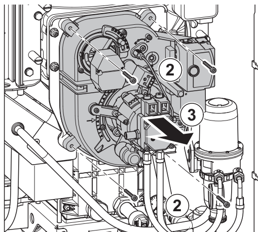
Fig.42 Retrait de la partie supérieure du brûleur
