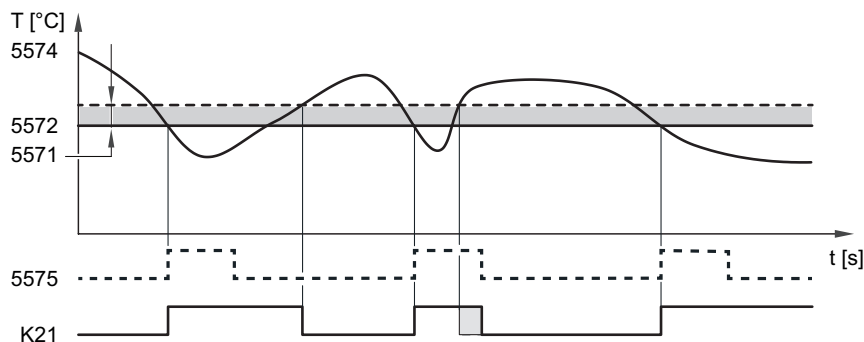
Fig.37 Surveillance de la température insuffisante
