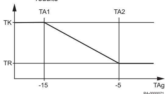
Fig.30 Augmentation de la consigne réduite
