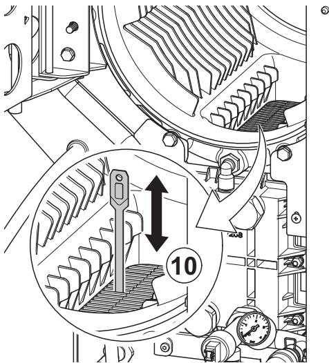
Fig.53 Nettoyage de l'échangeur thermique
