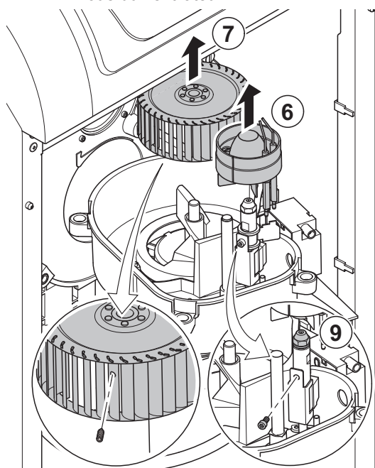
Fig.44 Démontage de l'unité de mélange/roue du ventilateur
