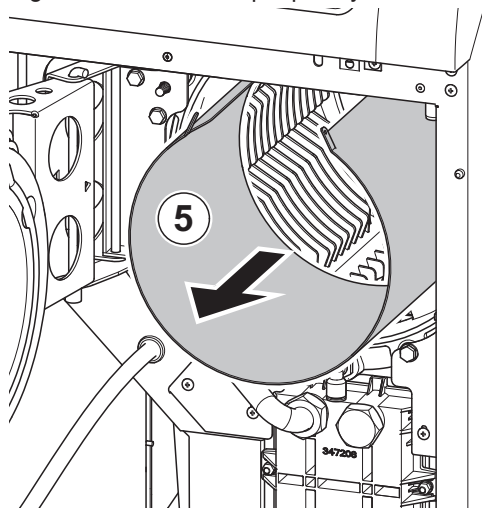
Fig.51 Retrait de la plaque foyère
