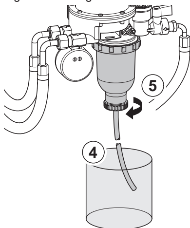
Fig.57 Retrait du filtre à fioul
