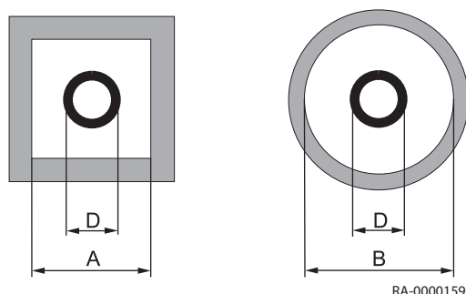
Fig.20 Dimensions minimales du conduit
