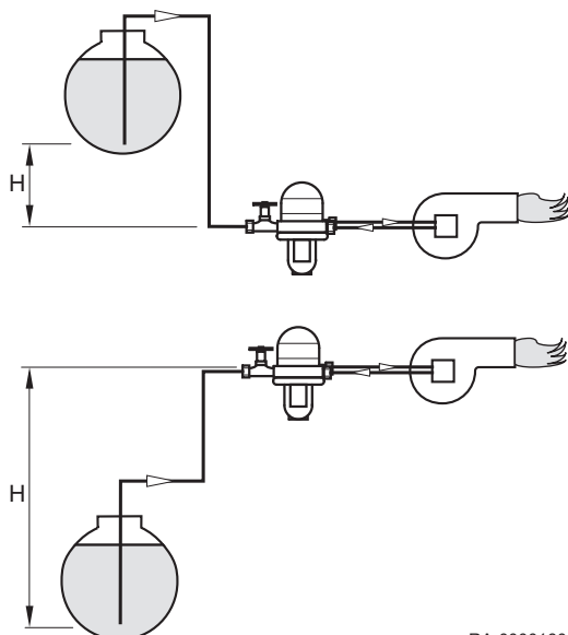
Fig.18 Système à une ligne avec filtre à fioul
