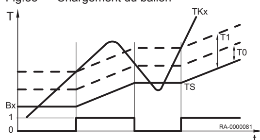
Fig.35 Chargement du ballon
