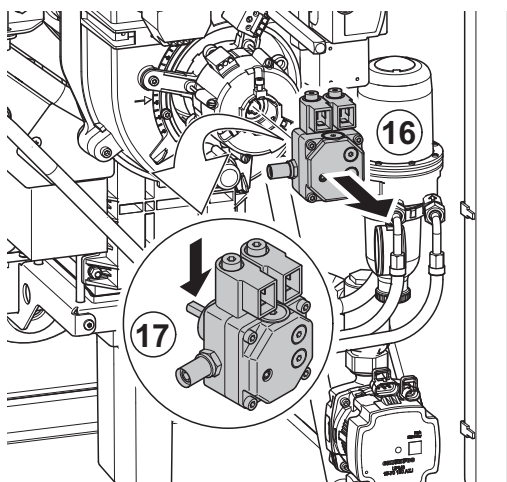
Fig.47 Dépose de la pompe à fioul
