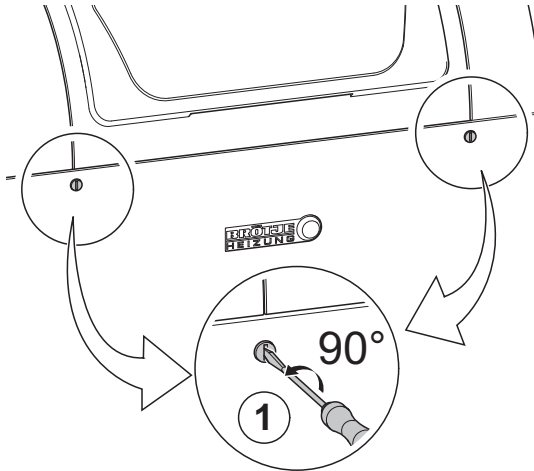
Fig.16 Desserrer les attaches rapides
