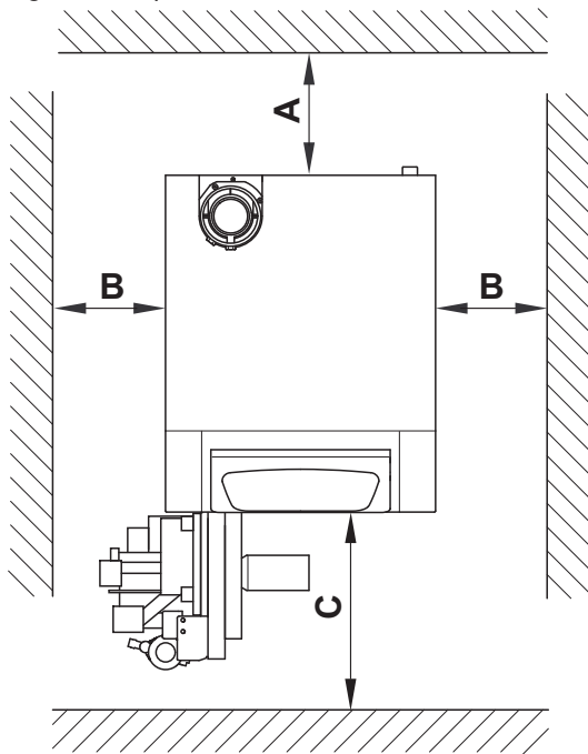
Fig.12 Espace nécessaire
