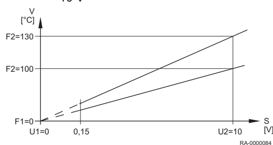
Fig.39 Exemple de demande de chaleur 10 V
