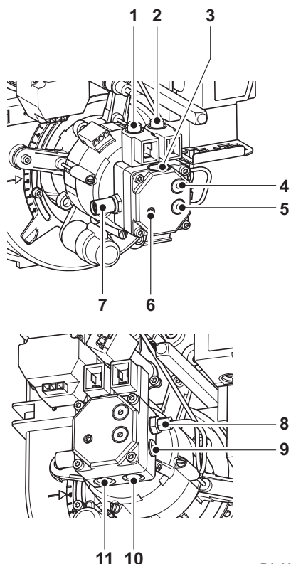
Fig.7 Éléments et connexions en fonctionnement
