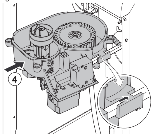
Fig.43 Position d'entretien
