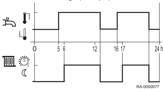
Fig.33 Déclenchement en fonction du programme de l'heure 4 (exemple)
