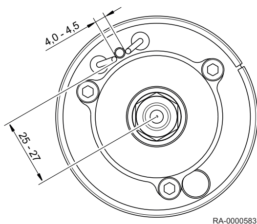
Fig.60 Dimensions de réglage
