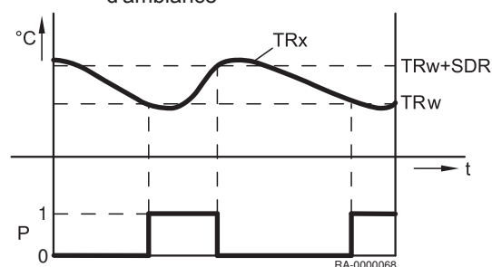
Fig.27 Limitation de la température d'ambiance
