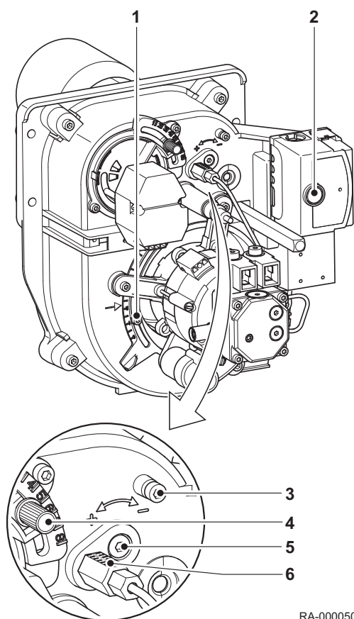
Fig.6 Touches du tableau de commande
