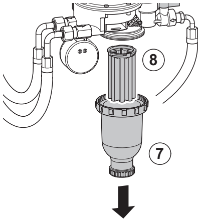
Fig.58 Remplacement de l'élément filtrant
