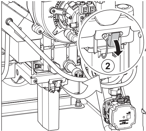
Fig.41 Retrait du siphon
