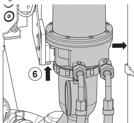
Fig.57 Retrait du filtre à fioul
