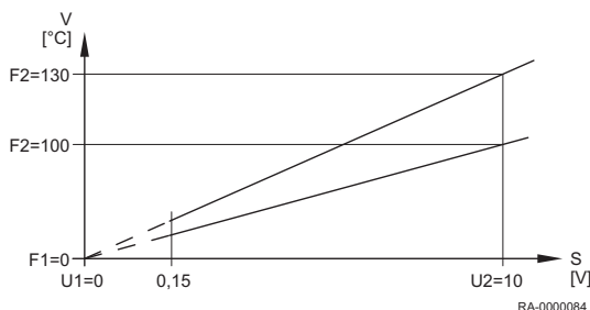
Fig.40 Exemple de demande de chaleur 10 V
