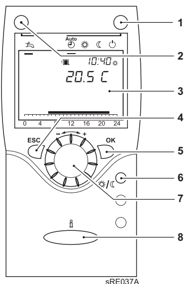
Fig.8 Interface de fonctionnement de l'appareil d'ambiance RGT
