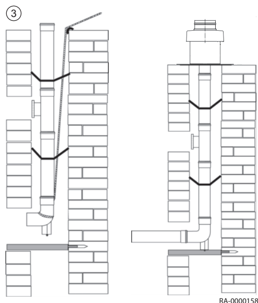
Fig.22 Insertion dans le conduit
