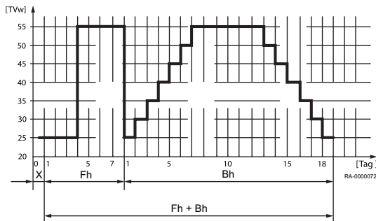
Fig.31 Profil de température de la fonction du durcissement de sol
