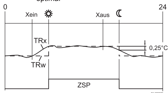
Fig.29 Commande de démarrage et d'arrêt optimal
