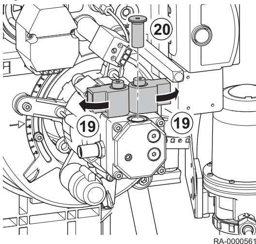
Fig.48 Retrait du filtre à fioul
