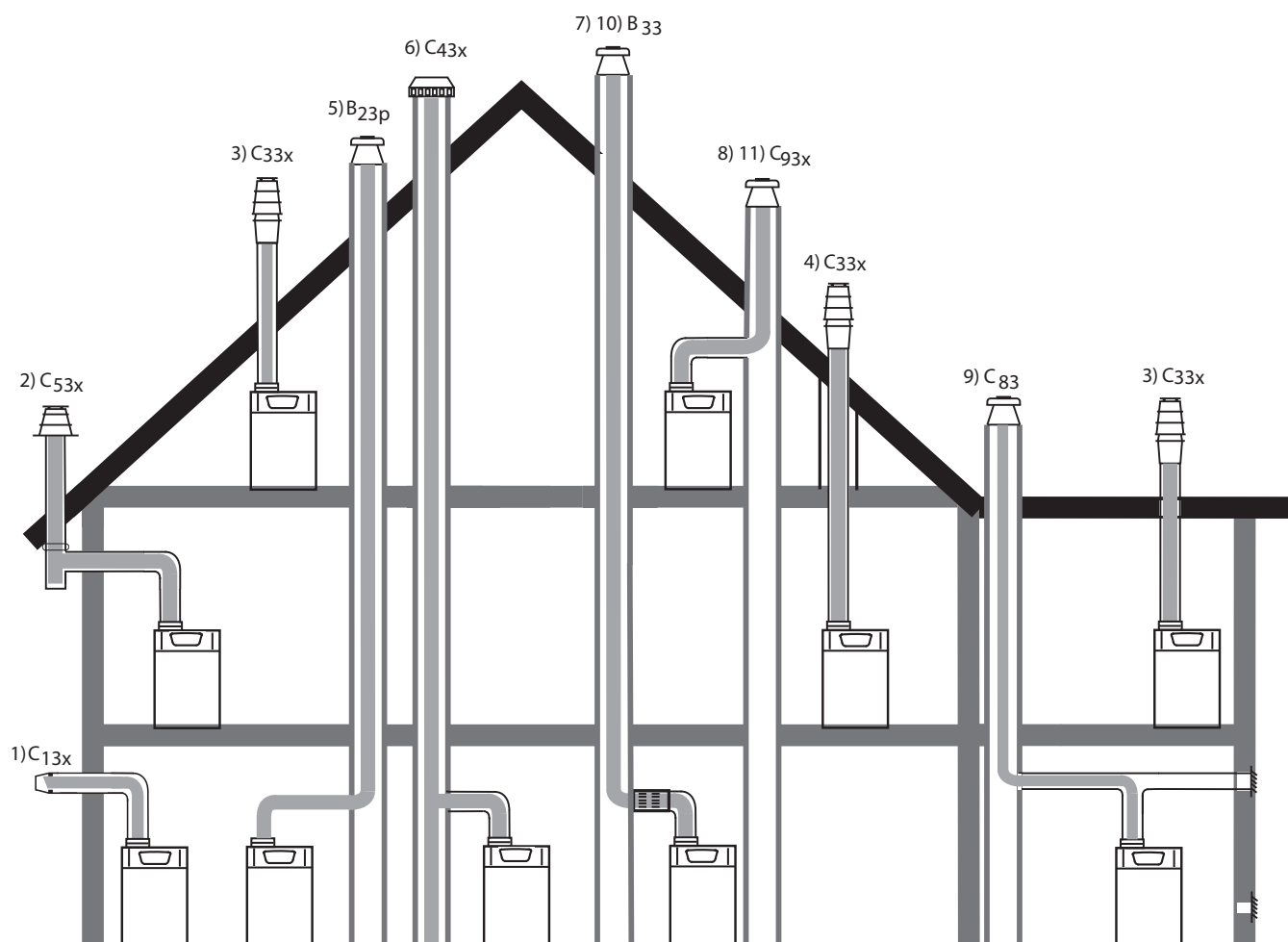
Fig.19 Options de raccordement avec KAS 80 (accessoires)
