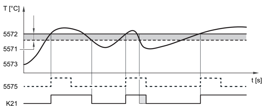
Fig.36 Surveillance de la température excessive
