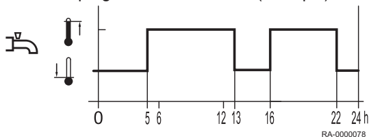
Fig.33 Déclenchement en fonction du programme de l'heure 4 (exemple)
