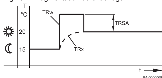
Fig.28 Augmentation du chauffage
