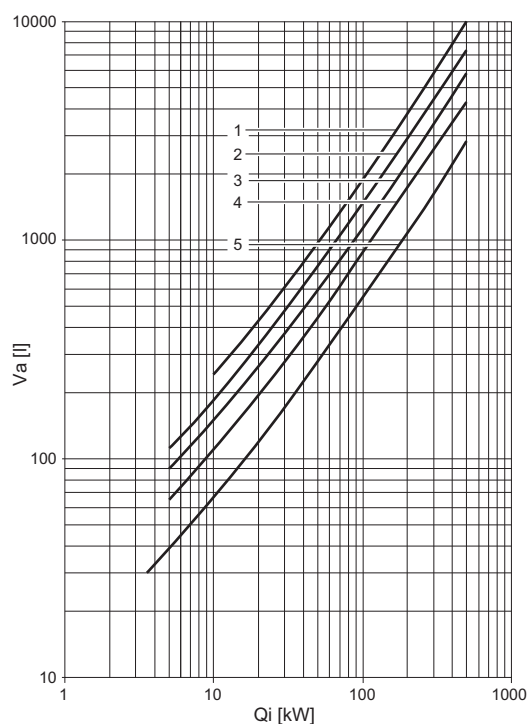
Fig.11 Détermination du volume de l'installation
