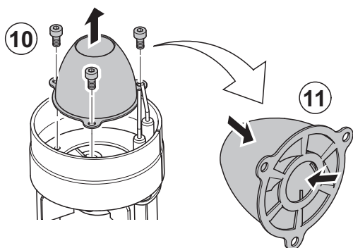
Fig.45 Retrait et nettoyage du gicleur d'air
