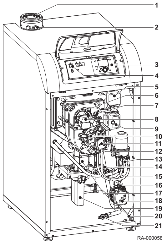
Fig.5 Vue de la chaudière
