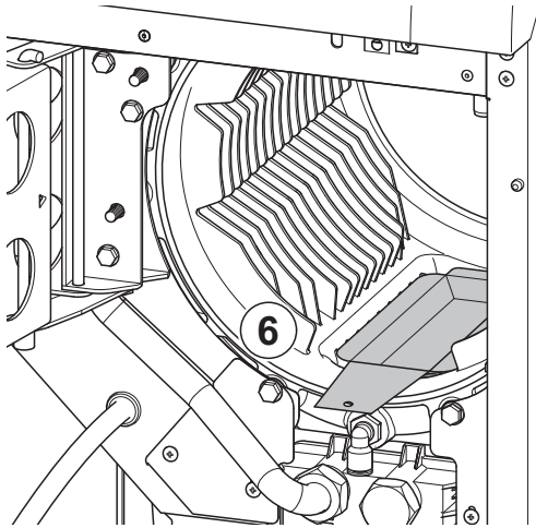
Fig.52 Insertion du plateau de nettoyage
