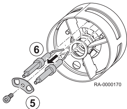
Fig.59 Retrait des électrodes d'allumage
