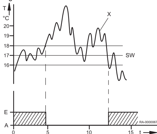
Fig.26 Limite chauffe été/hiver
