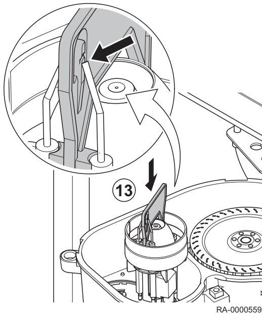
Fig.47 Dépose de la pompe à fioul
