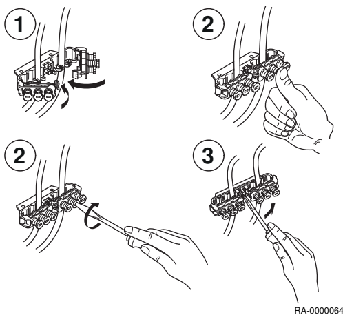
Fig.23 Arrêts de traction
