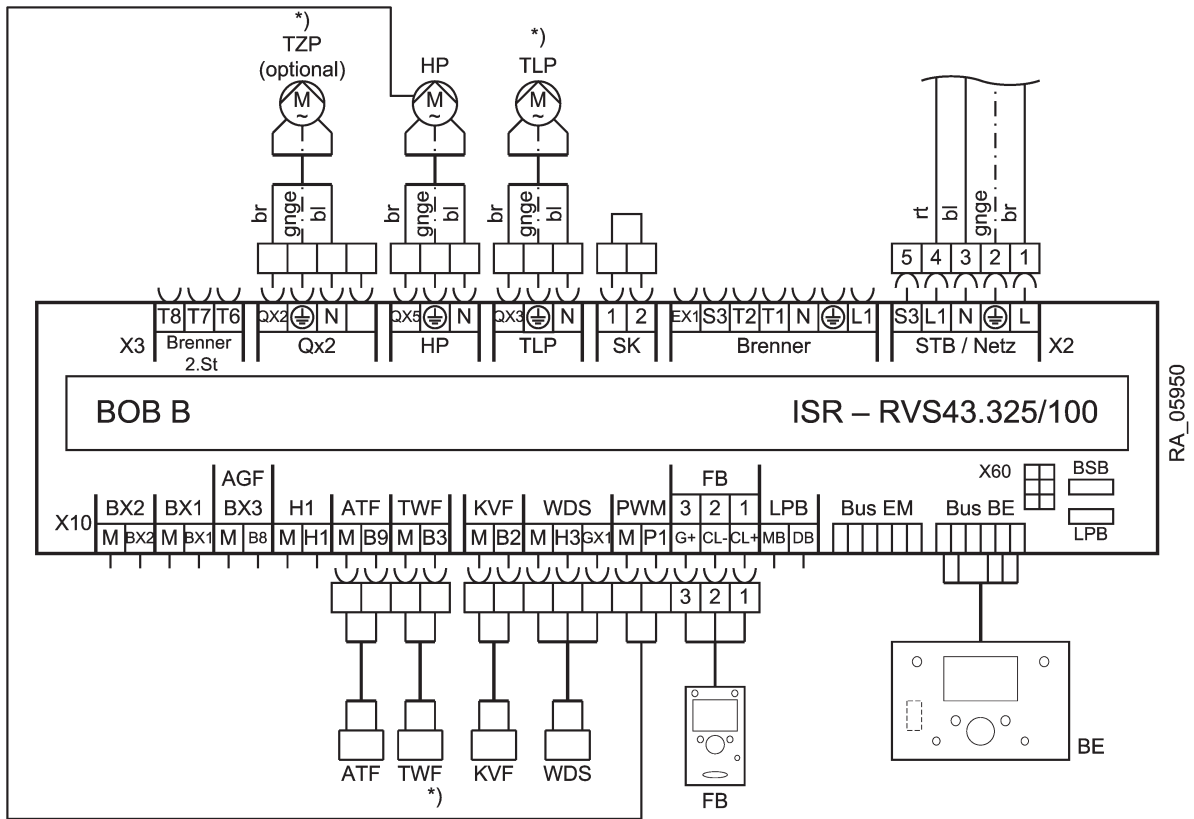
Fig.15 Schéma de câblage – BORA EVO HTE, un circuit de chauffage à pompe avec appareil d'ambiance, y compris commande de la température du ballon
