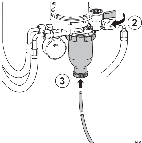
Fig.56 Vidange du fioul
