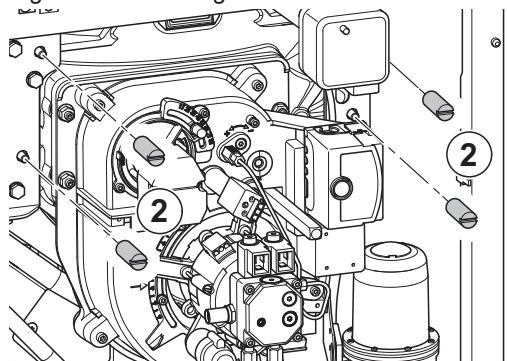
Fig.49 Démontage des écrous de fixation
