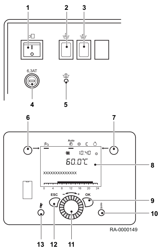
Fig.9 Description des touches
