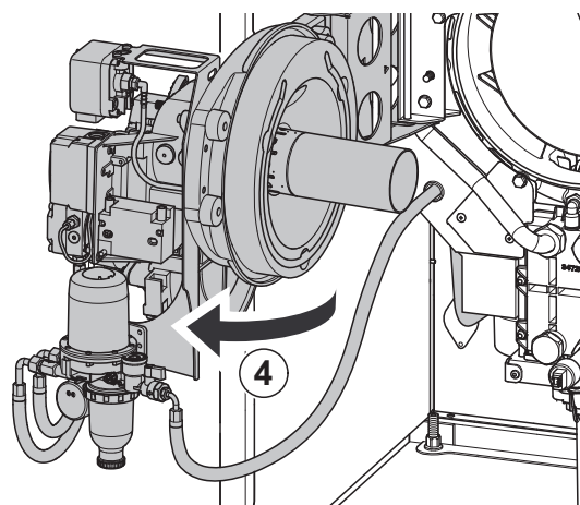
Fig.50 Extraction de la porte du brûleur
