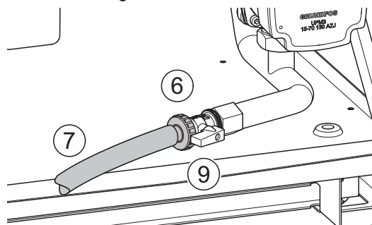
Fig.66 Robinet de remplissage et de vidange avec embout du flexible
