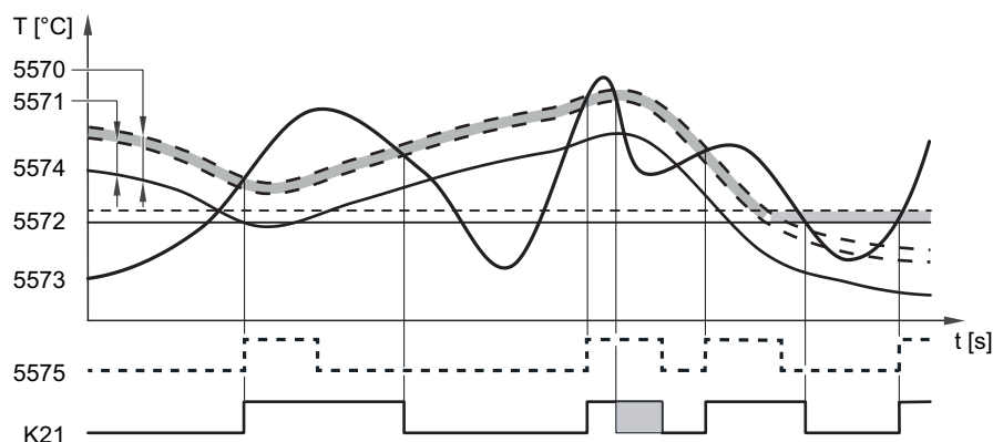
Fig.38 Variante d'utilisation Contrôleur de température différentielle
