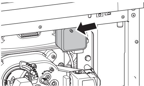
Fig.64 Bouton de déverrouillage du pressostat air
