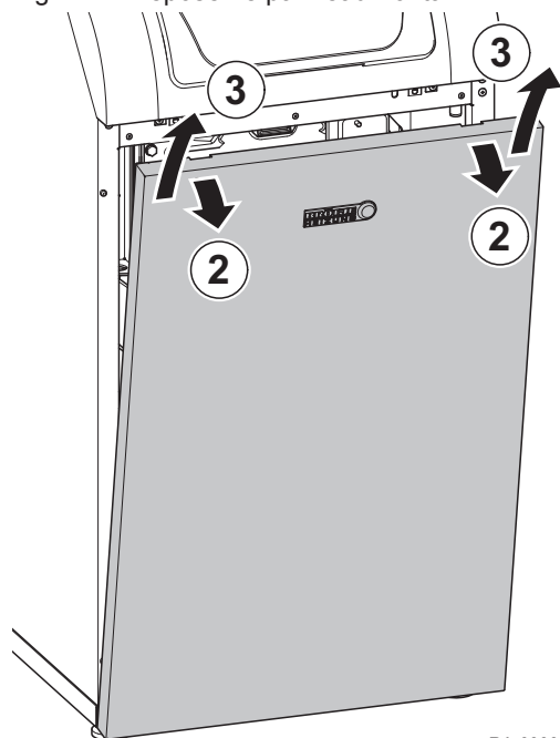
Fig.17 Déposer le panneau frontal
