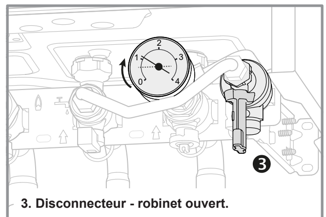
figure 5 - Remise en pression du circuit chauffage
