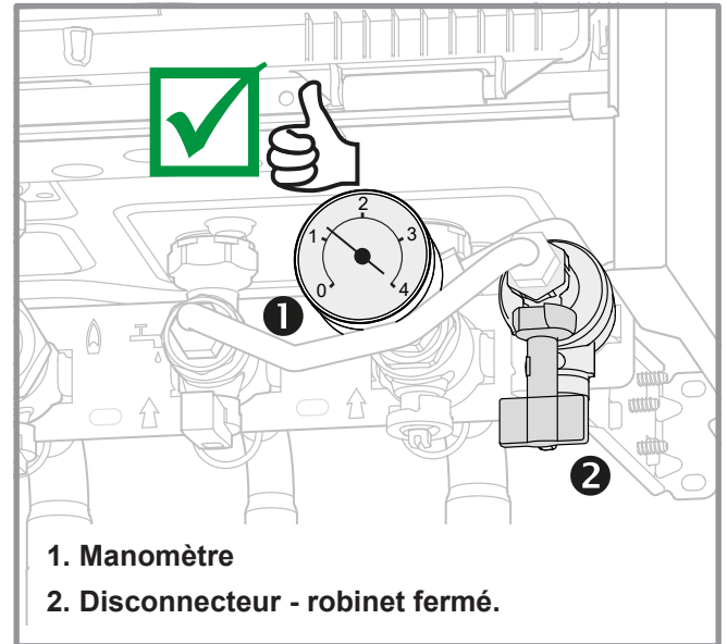
figure 3 - Contrôle de la pression hydraulique
