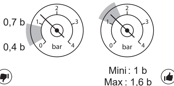
fig. 4 - Plages de pression
