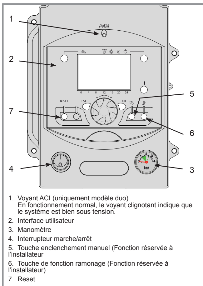
figure 56 - Tableau de contrôle
