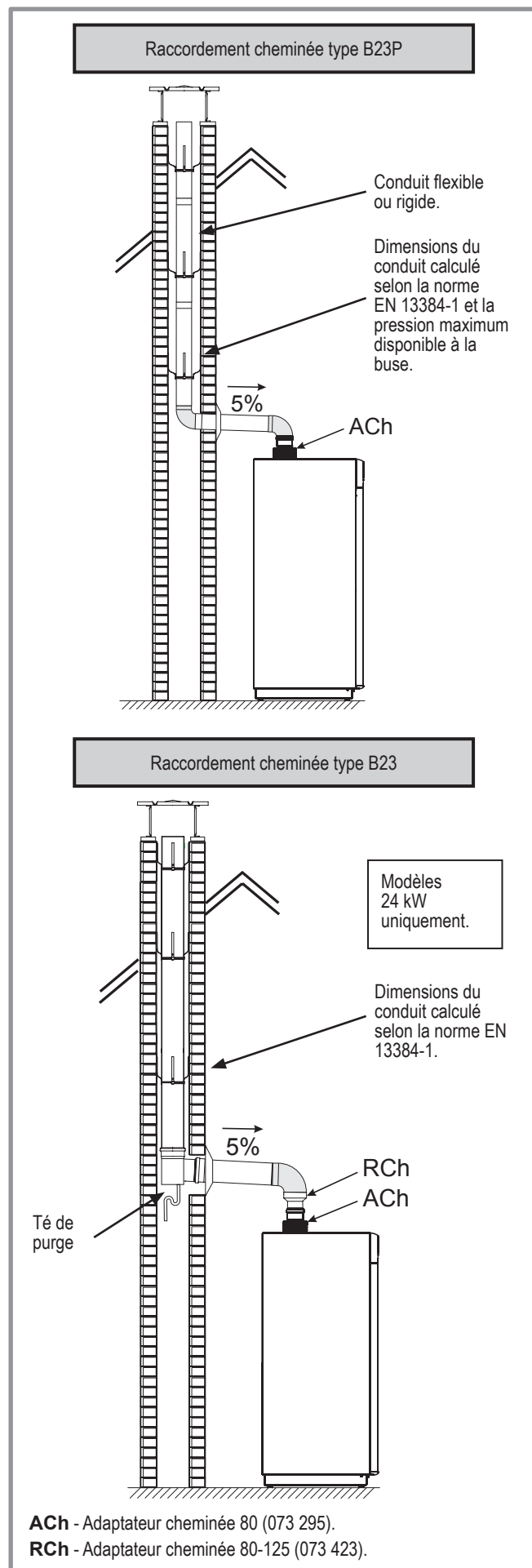
figure 20 - Possibilités de raccordement (type B23 et B23P)
