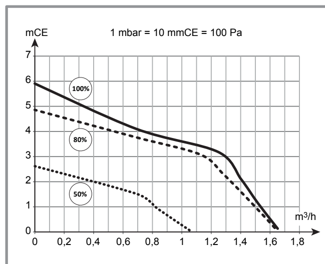
figure 5 - Pressions et débits disponibles 1 circuit (effinox condens duo 5024)
