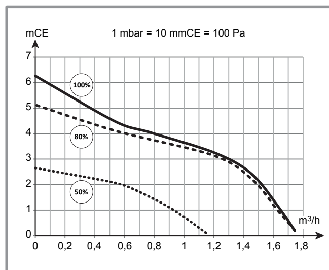
figure 7 - Pressions et débits disponibles 1 circuit (effinox condens duo 5030 / 5034)
