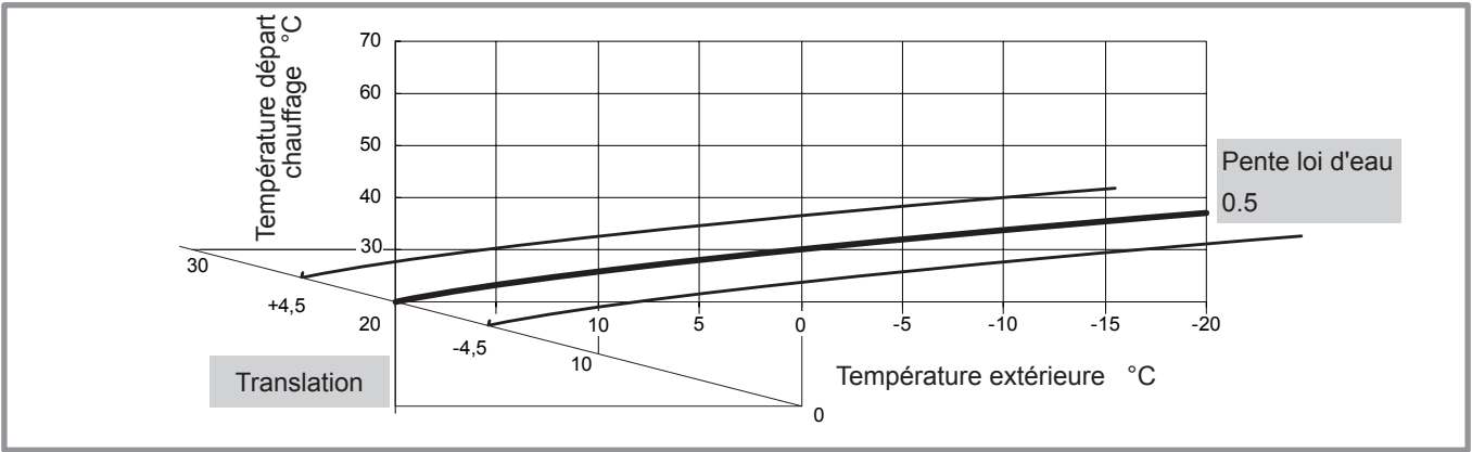
figure 46 - Translation de la courbe de chauffe (ligne 721)
