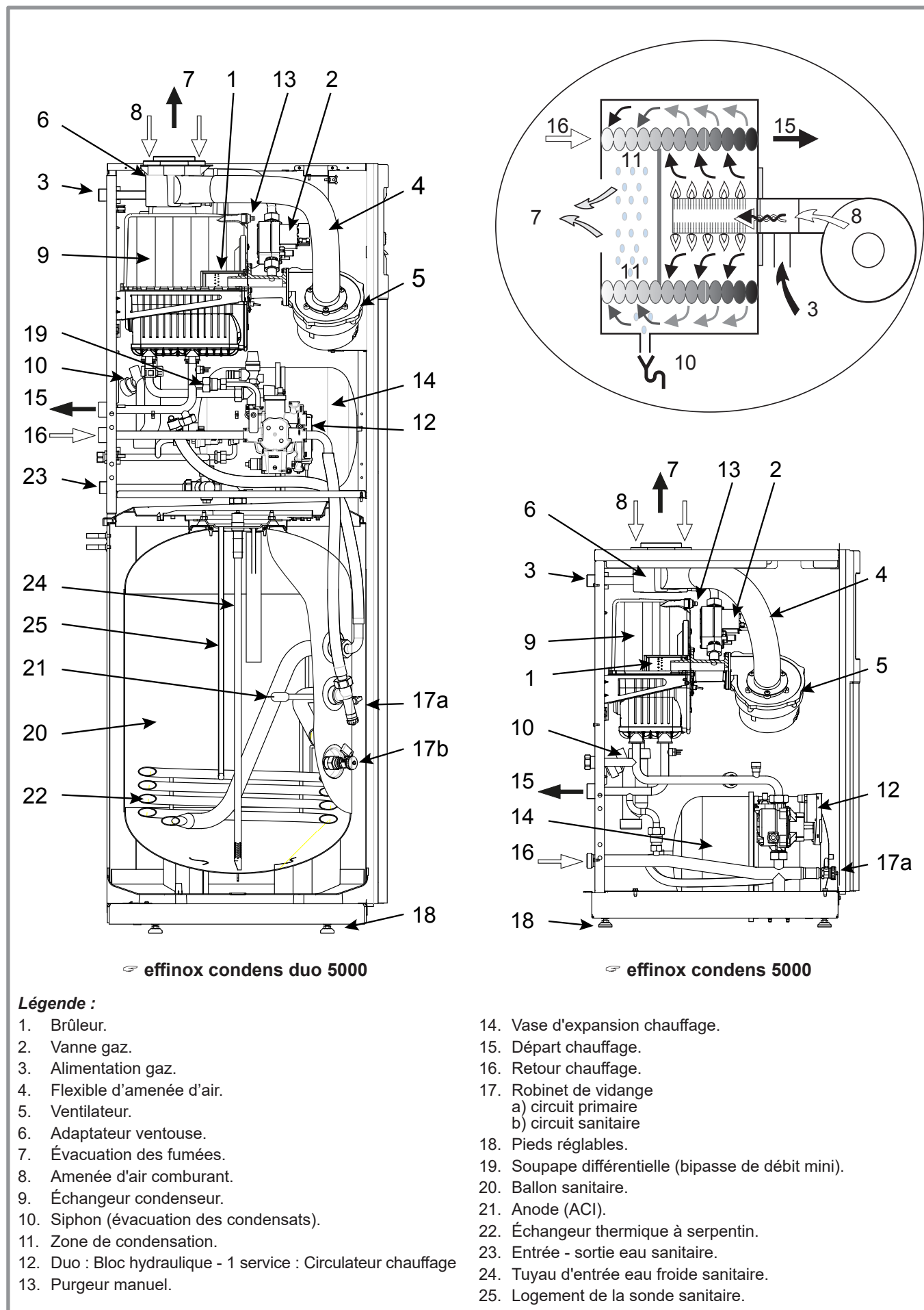
figure 8 - Coupe schématique de l'appareil
