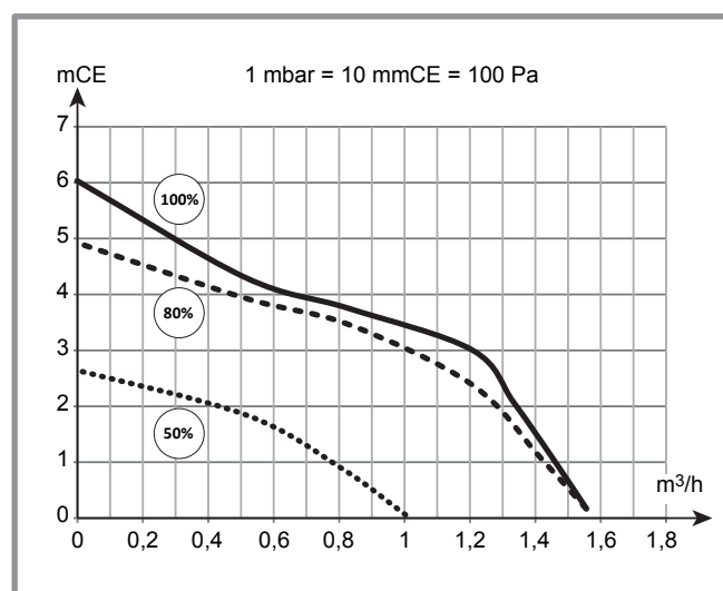
figure 5 - Pressions et débits disponibles 1 circuit (effinox condens duo 5022)
