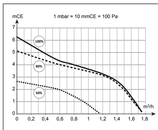
figure 6 - Pressions et débits disponibles 1 circuit (effinox condens duo 5030)
