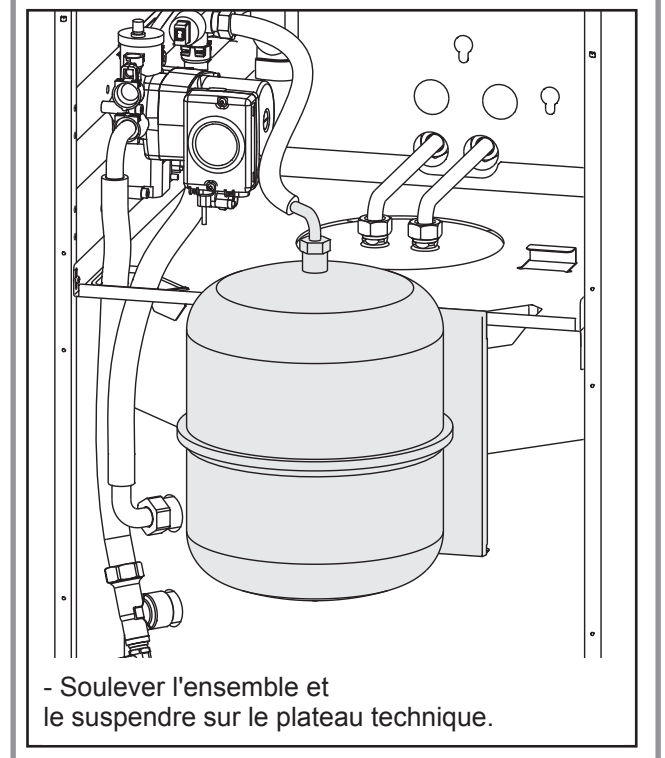
figure 44 - Accès au plateau technique (perfinox condens duo)
