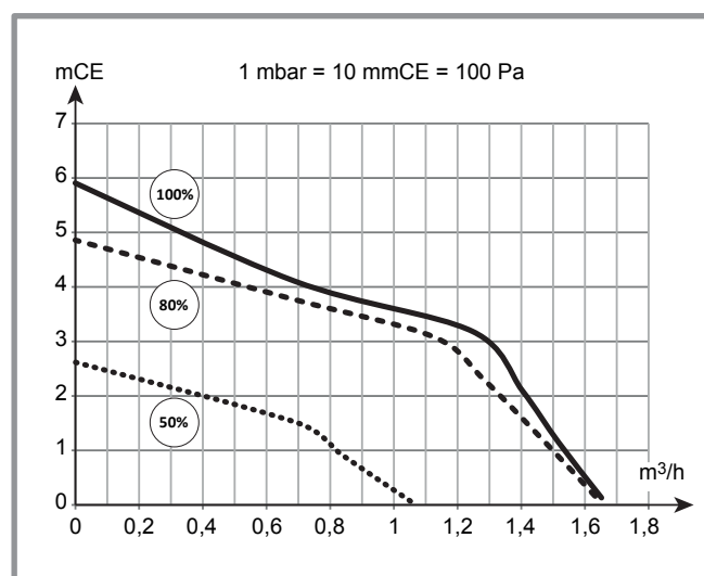
figure 5 - Pressions et débits disponibles perfinox condens duo 5028
