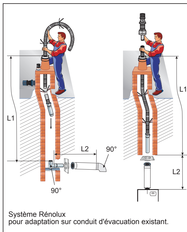
figure 12 - Possibilités de raccordement (type C13 et C33)
