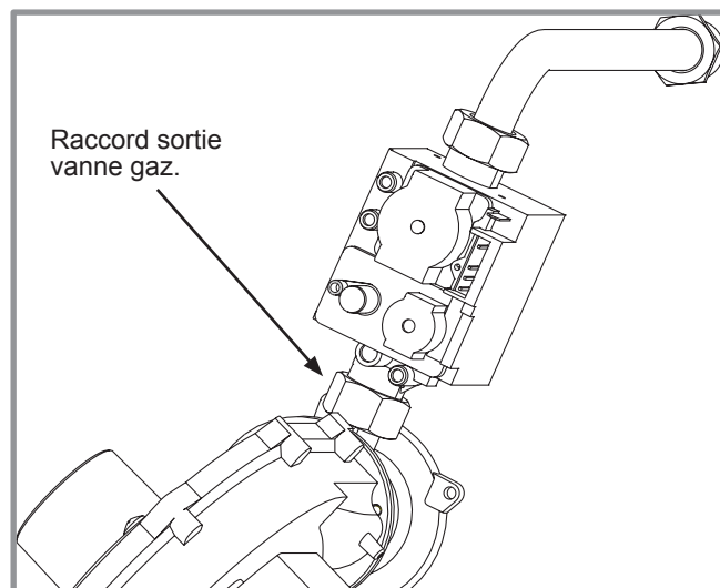
figure 18 - Accès au diaphragme
