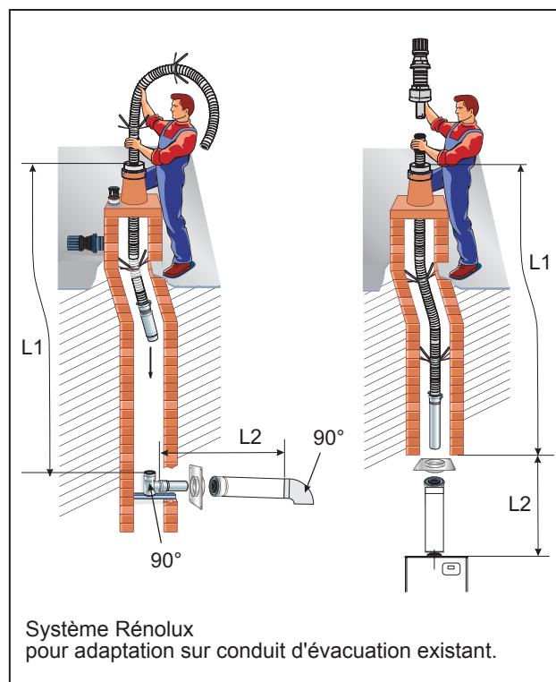
figure 21 - Possibilités de raccordement (type C13 et C33)
