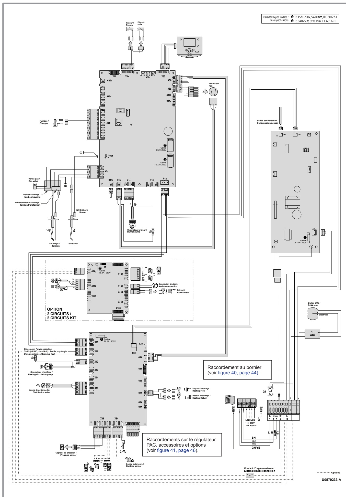
figure 55 - Câblage électrique module hydraulique (hors raccordements installateur)
