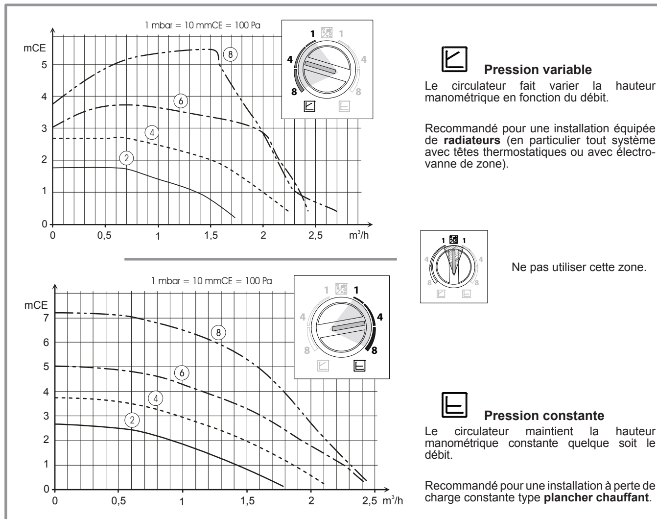
figure 42 - Pressions et débits hydrauliques disponibles
