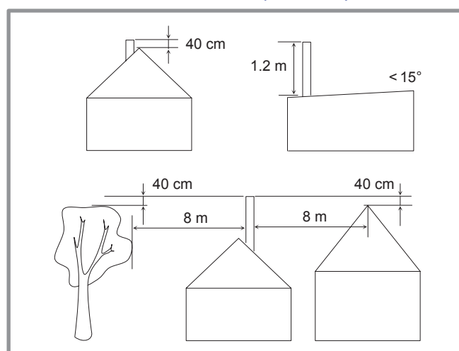
figure 19 - Hauteur de la souche du conduit d'évacuation (B23, B23P)
