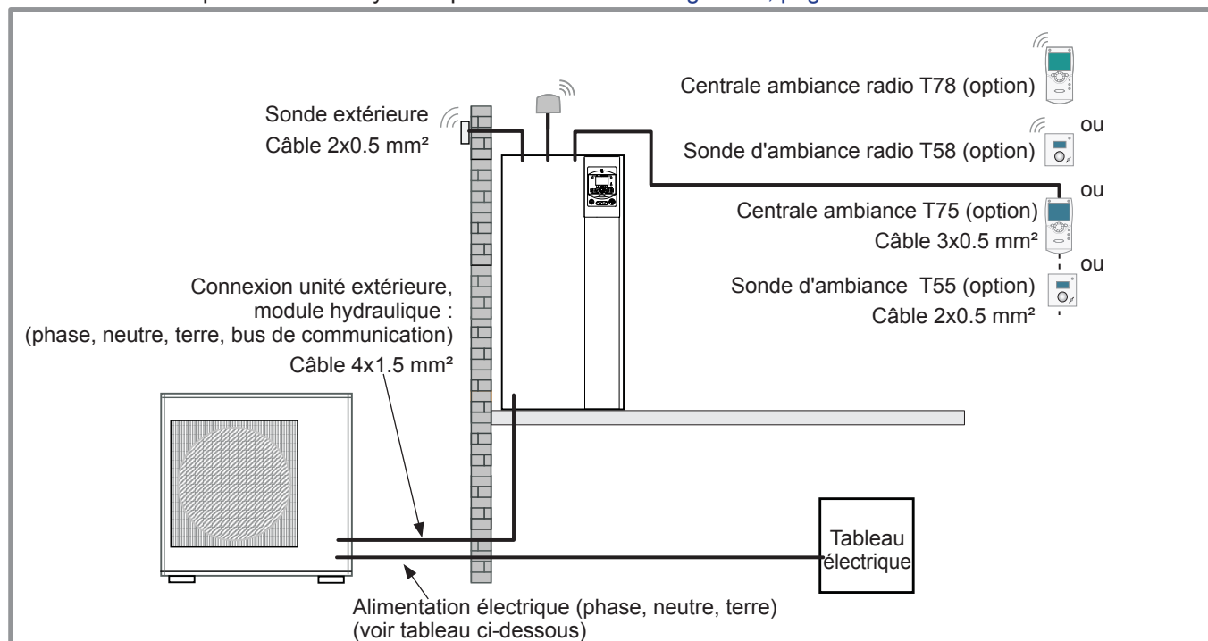
figure 36 - Schéma d'ensemble des raccordements électriques pour une installation simple (1 circuit de chauffe)
