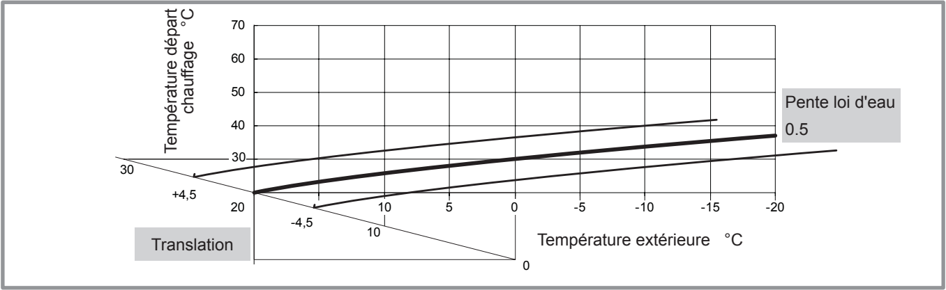
figure 51 - Translation de la courbe de chauffe (ligne 1021)
