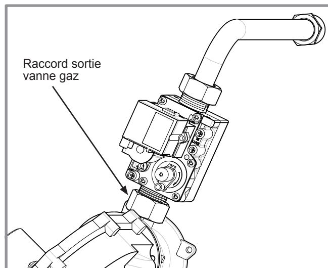
figure 34 - Accès au diaphragme
