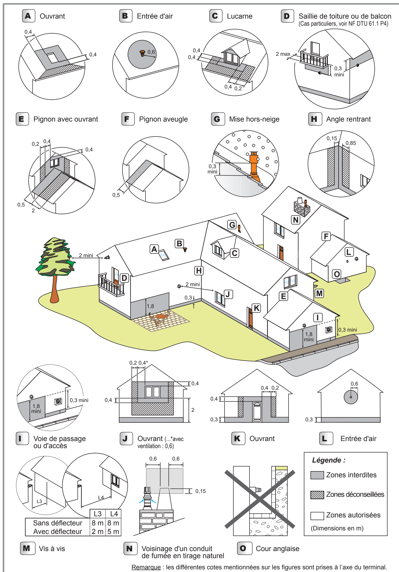
figure 23 - Règles d'implantation du terminal pour chaudières gaz étanches (C13, C33, C53)
