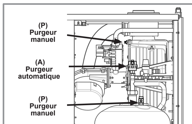
figure 32 - Purgeurs du module hydraulique
