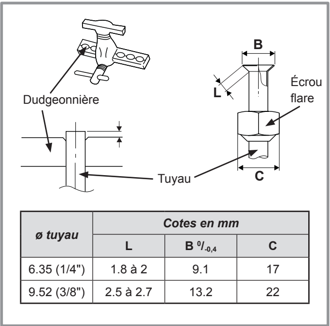
figure 24 - Evasement pour liaisons flare
