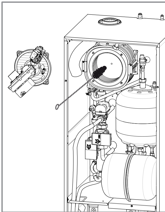
figure 56 - Accès à la chambre de combustion
