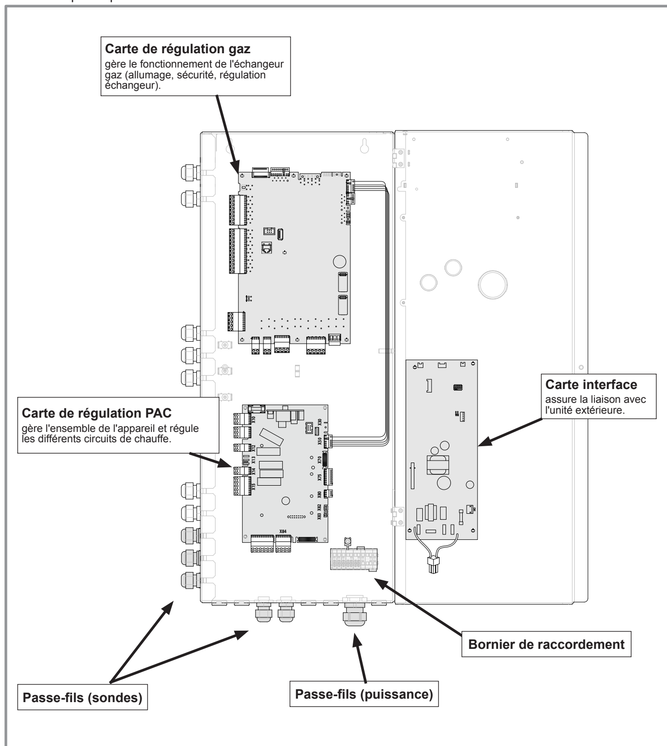
figure 39 - Descriptif du coffret électrique du module hydraulique
