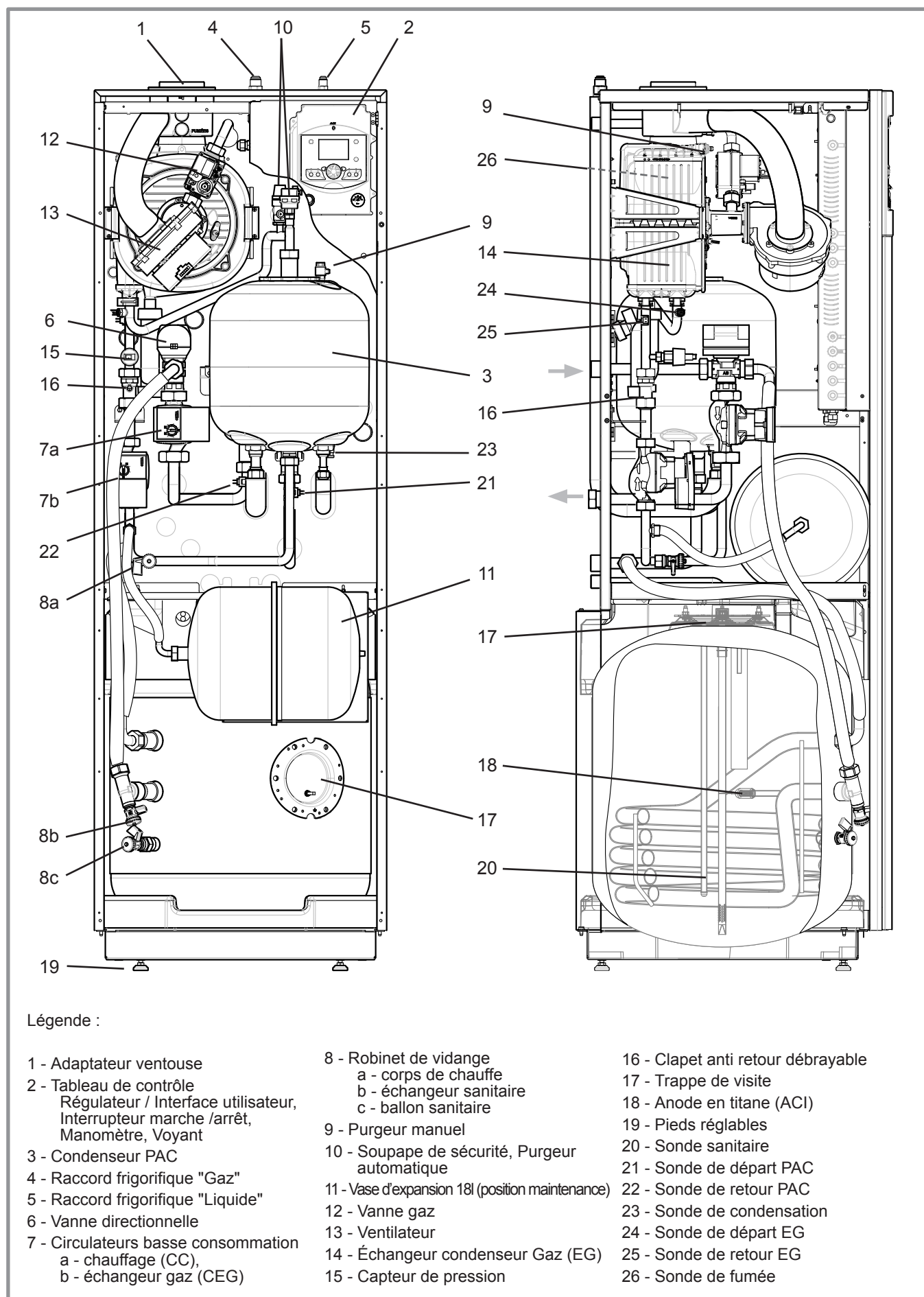
figure 6 - Organes du module hydraulique
