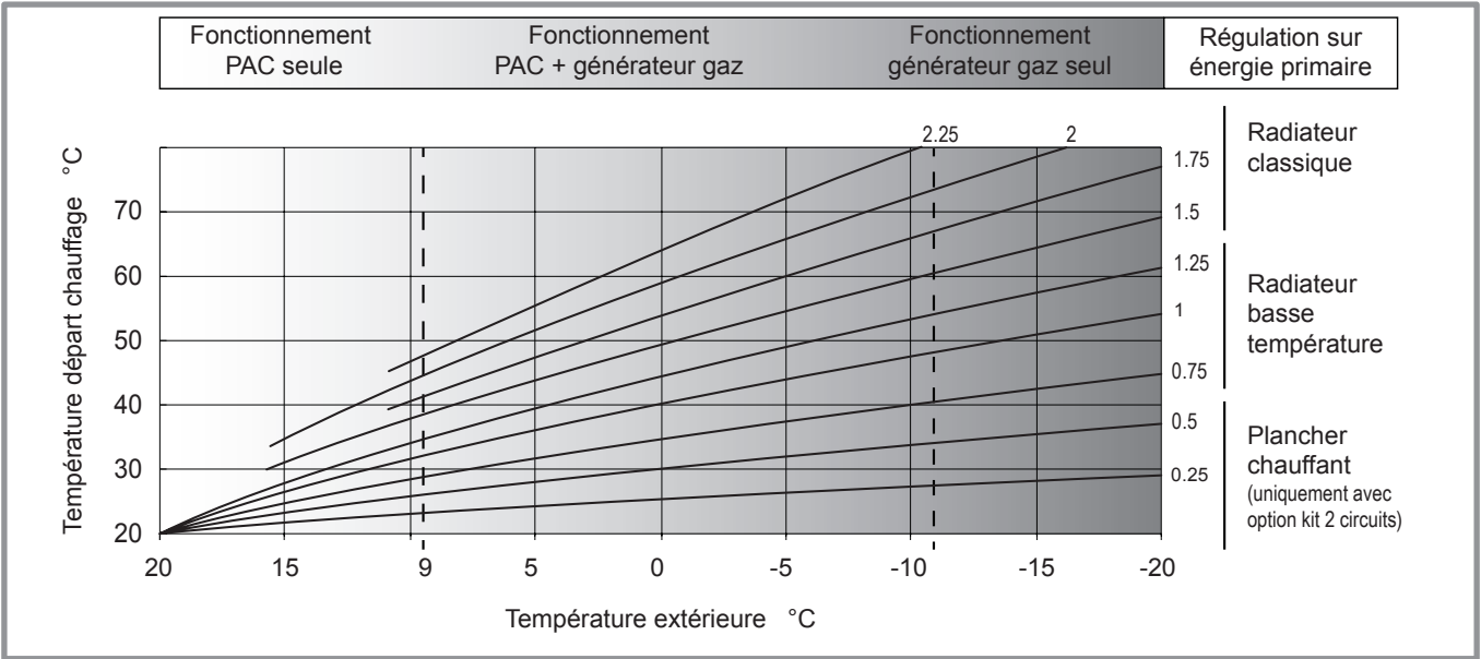
figure 50 - Pente de la courbe de chauffe (ligne 1020)
