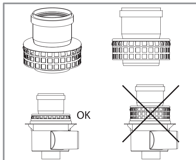
figure 18 - Montage de l'adaptateur cheminée 073295 (B23, B23P)
