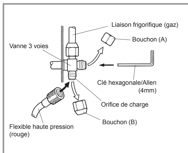
figure 28 - Raccordement du flexible sur la vanne gaz
