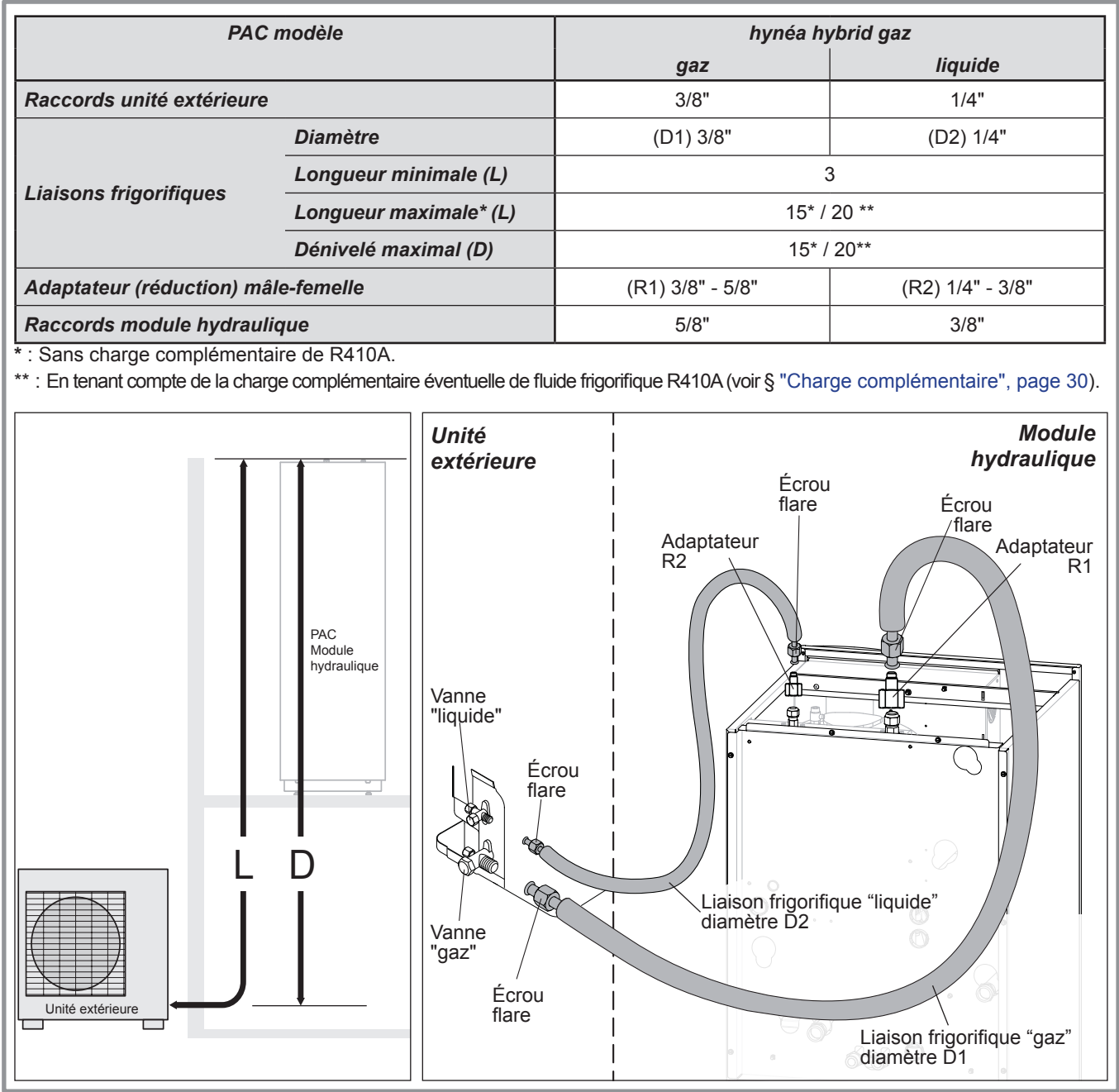
figure 27 - Raccordement des liaisons frigorifiques (diamètres et longueurs permises)
