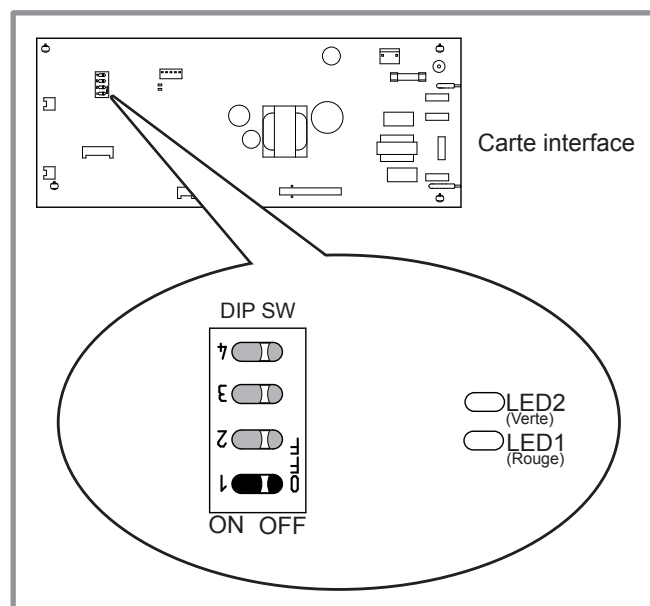
figure 30 - Emplacement des interrupteurs DIP et des diodes sur la carte d'interface du module hydraulique
