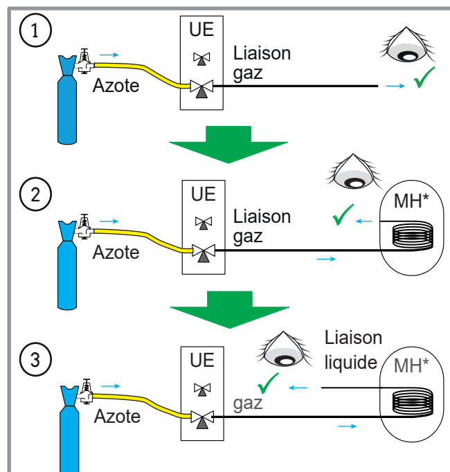
figure 26 - Vérification des liaisons frigorifiques
