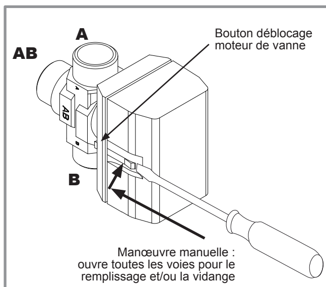
figure 60 - Position intermédiaire de la vanne directionnelle
