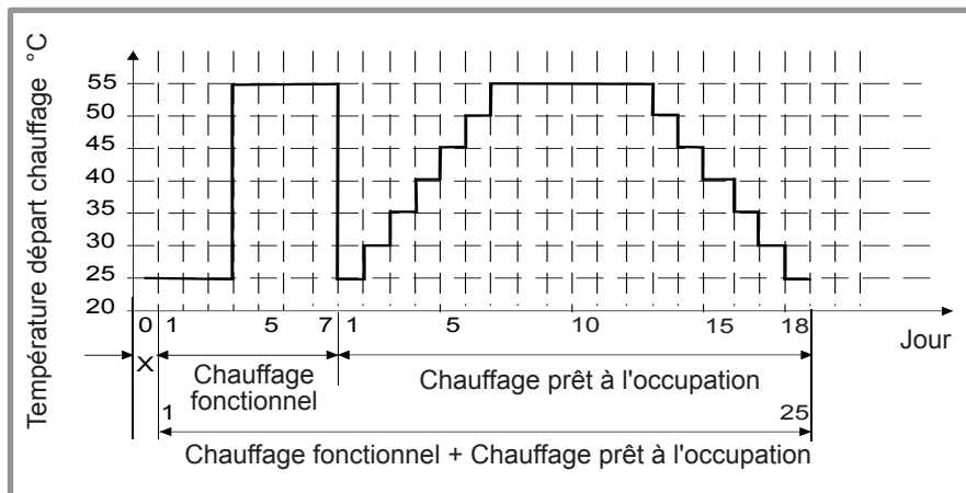
figure 53 - Diagramme des programmes de séchage de dalle
