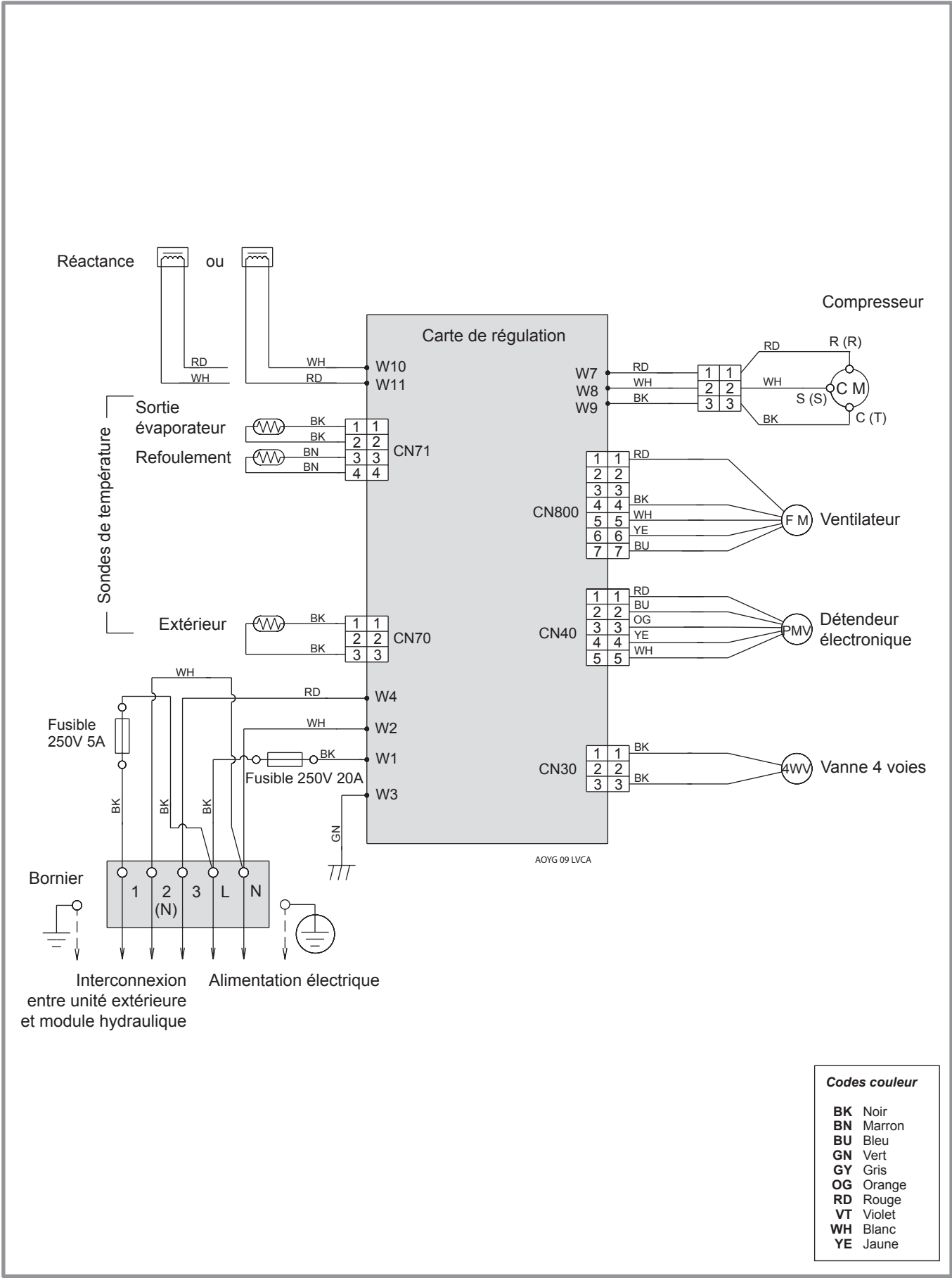
figure 54 - Câblage électrique unité extérieure modèle hynéa hybrid duo gaz (AOYG 09 LVCA)
