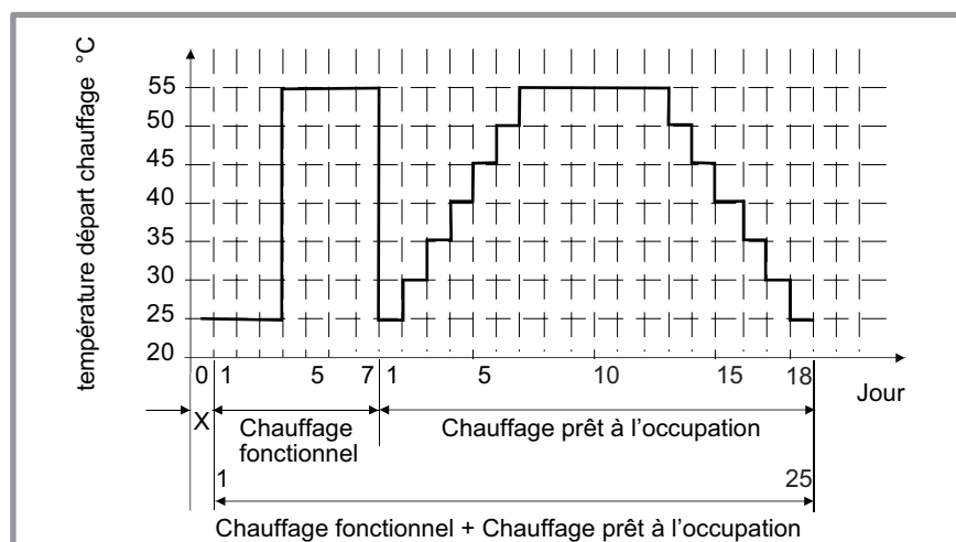
fig. 46 - Diagramme des programmes de séchage de dalle
