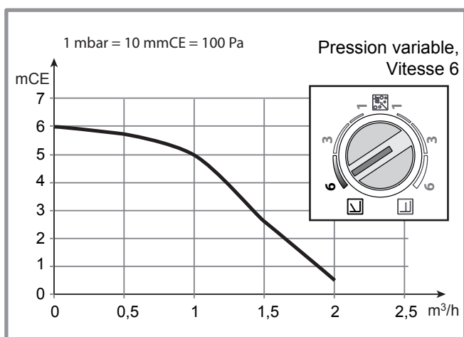
fig. 5 - Pressions et débits hydrauliques disponibles axe condens duo 5025 et 5032- 1 circuit
