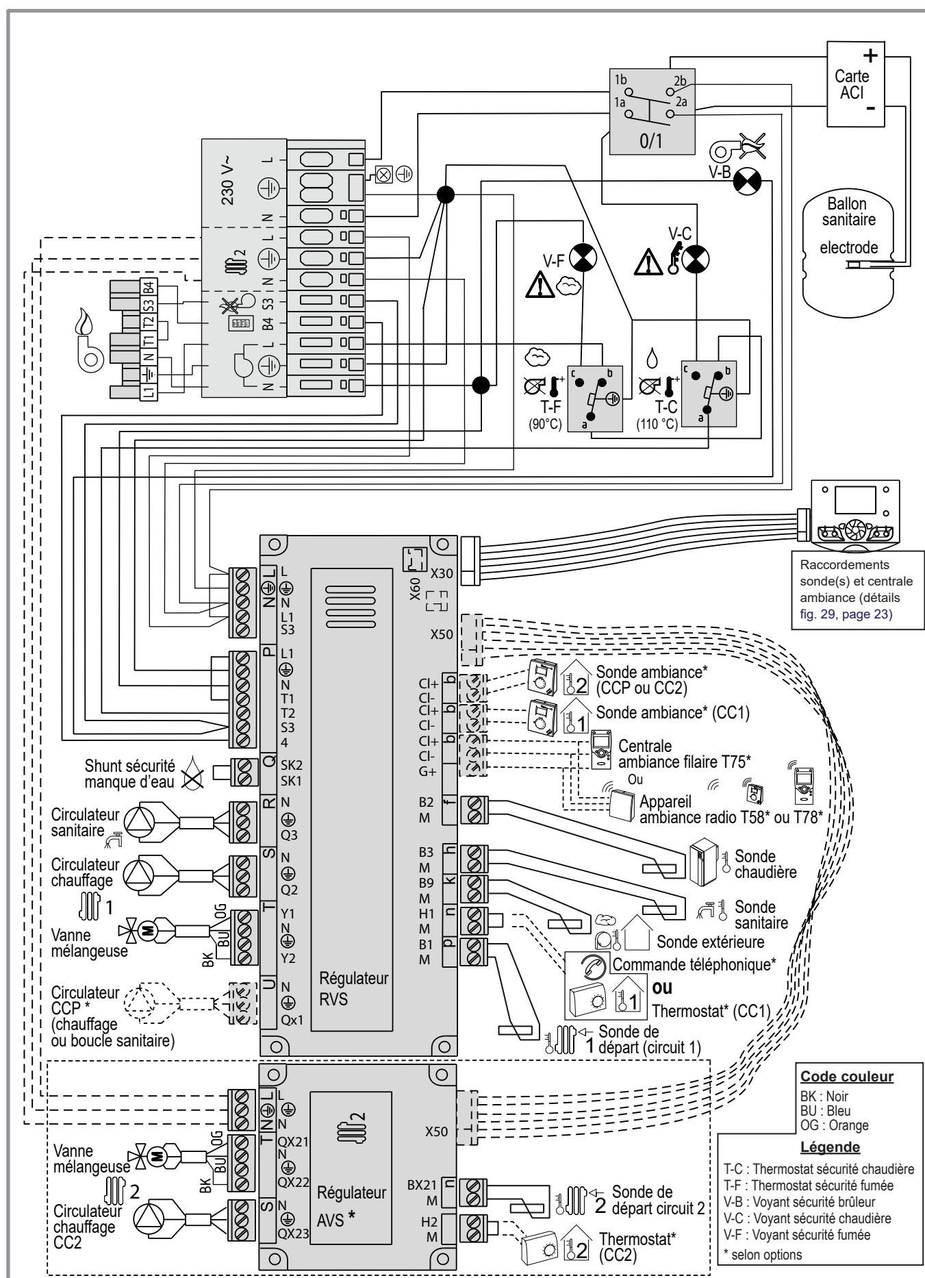
fig. 48 - Câblage électrique
