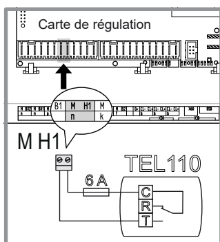
fig. 25 - Commande téléphonique
