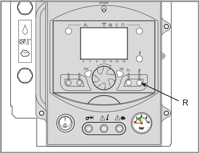
fig. 34 - Tableau de contrôle et régulation
