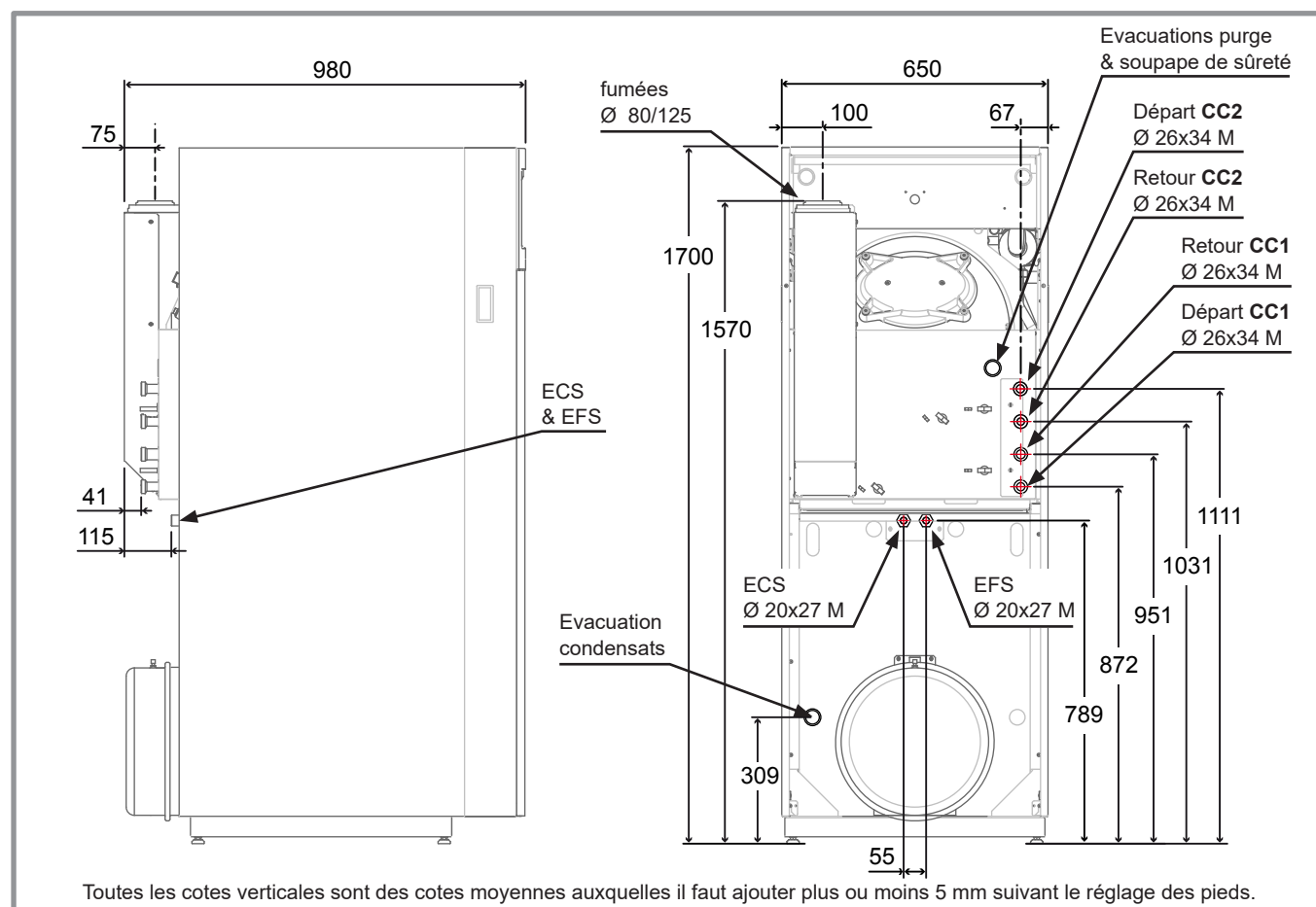
fig. 2 - Dimensions axeo condens duo en mm (avec kit hydraulique 2 circuits)
