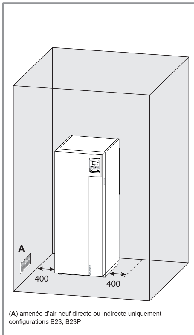
fig. 13 - Dégageurs minimum d'installation autour de la chaudière
