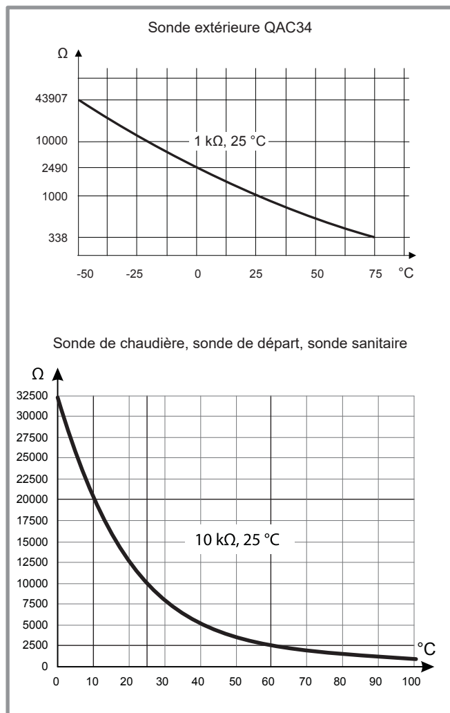
fig. 3 - Valeur ohmique des sondes
