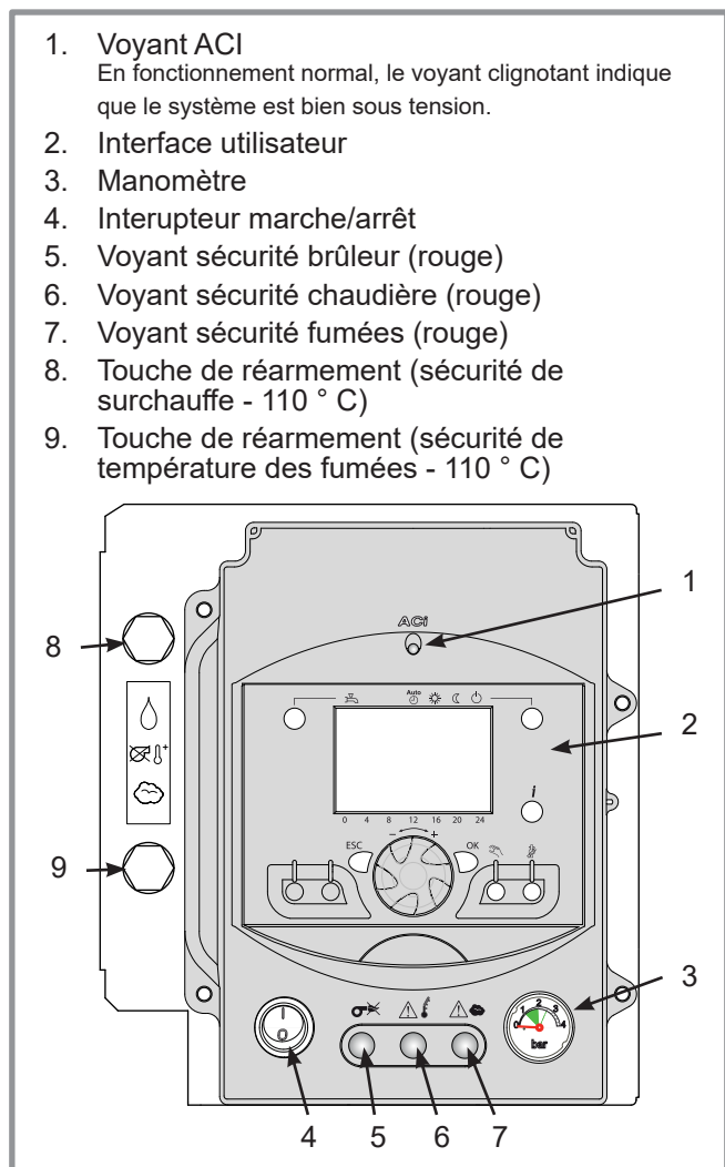
fig. 50 - Tableau de contrôle et régulation
