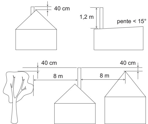
fig. 15 - Hauteur de la souche du conduit d'évacuation (B23P)
