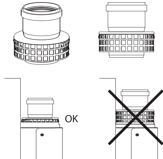
fig. 16 - Montage de l'adaptateur cheminée 073295 (B23, B23P)
