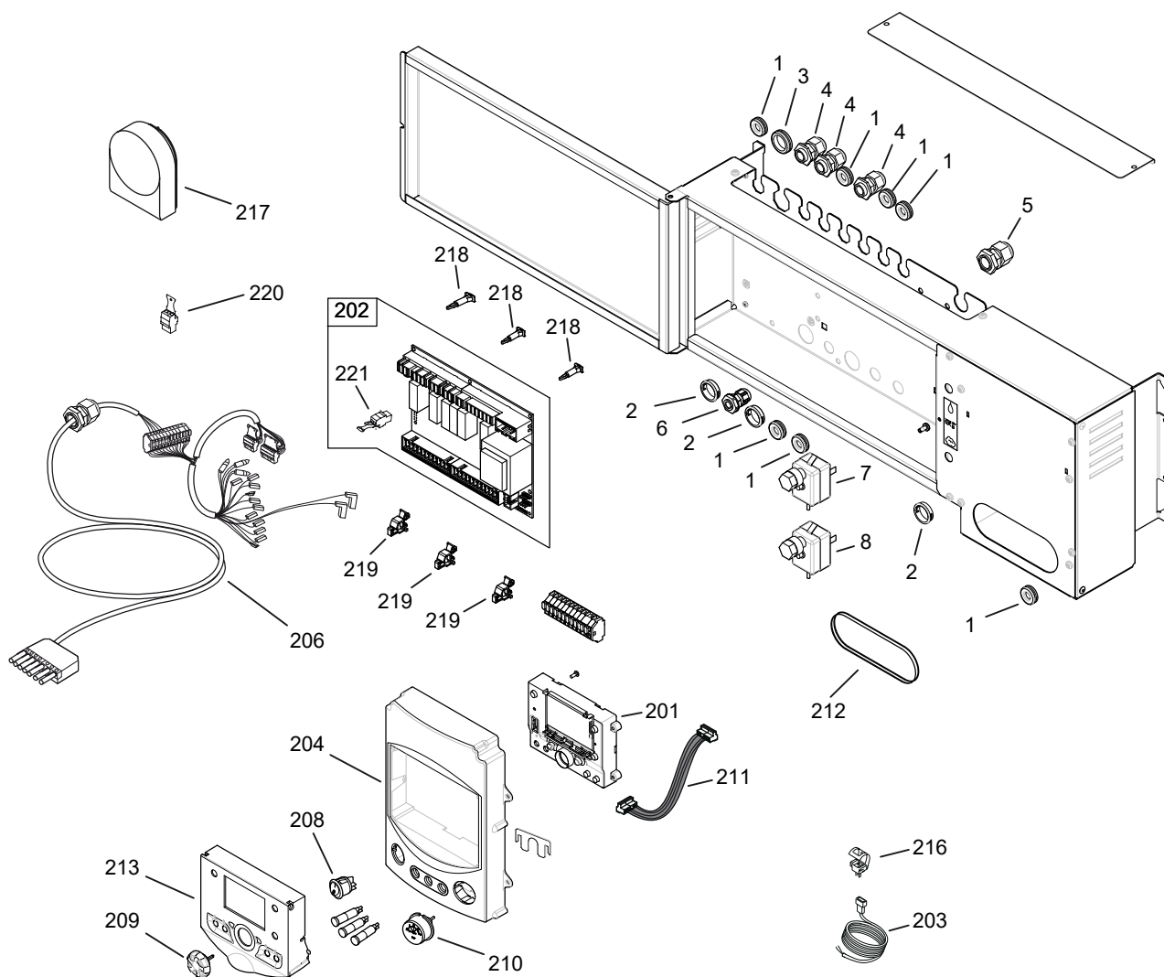
fig. 40 - Vue éclatée (tableau de contrôle)
