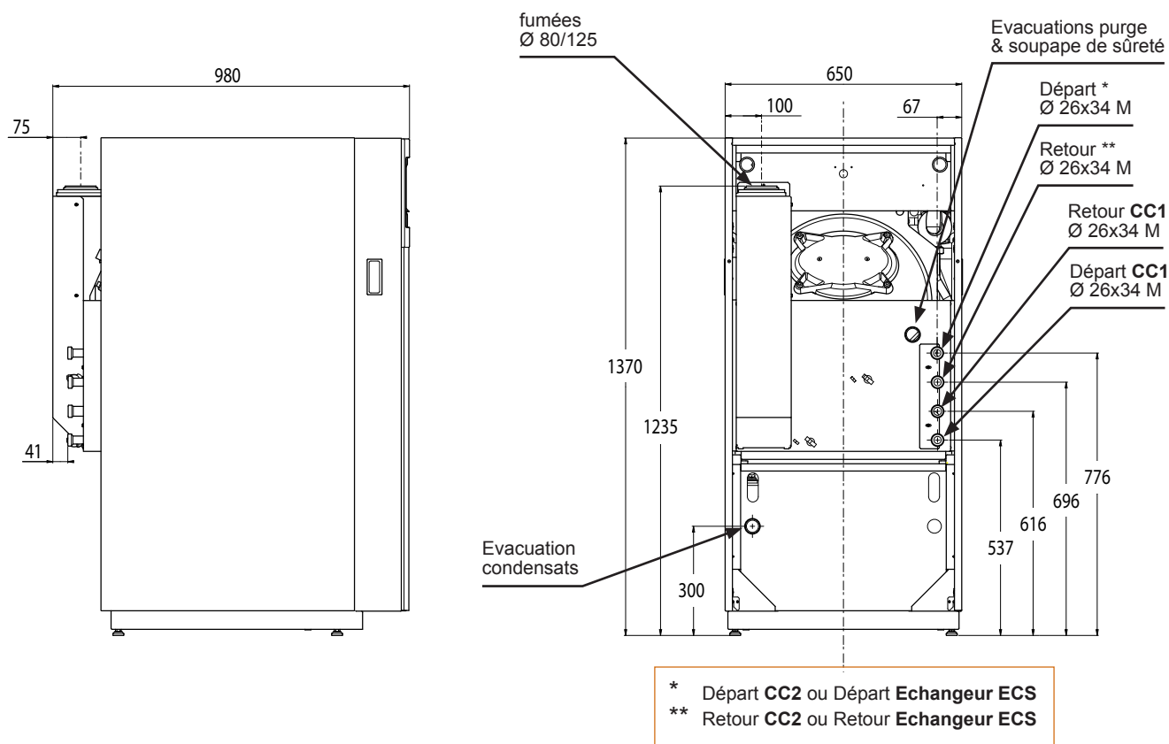
fig. 2 - Dimensions axexo nox en mm (* avec kit hydraulique 2 circuits ou ** avec kit sanitaire)
