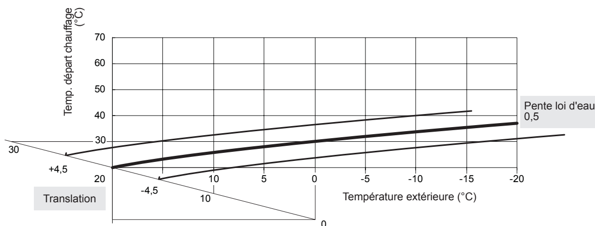
fig. 36 - Translation de la courbe de chauffe (ligne 721)
