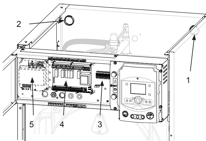
fig. 27 - Connecteur régulation
