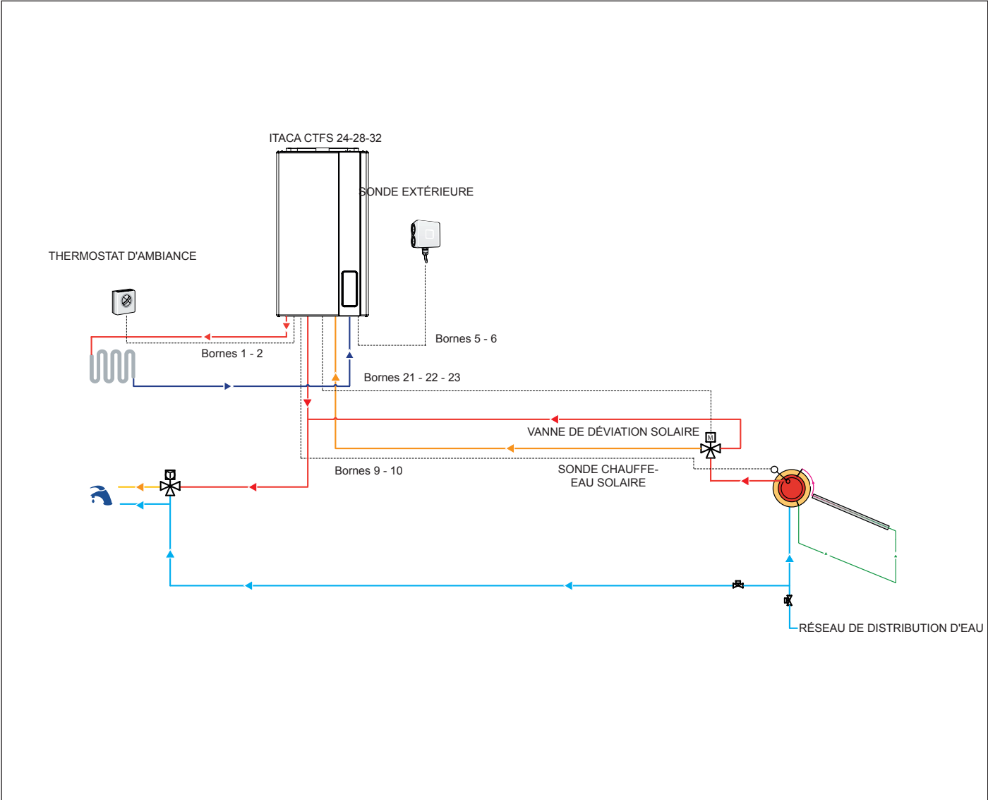
Fig. 14 Schéma de raccordement installation solaire à circulation naturelle avec chaudière combinée
