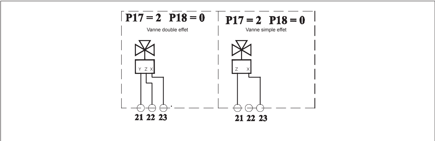
Fig. 15 Schéma de raccordement relais multifonction (X= neutre ; Y= dans la chaudière ; Z= au collecteur)
