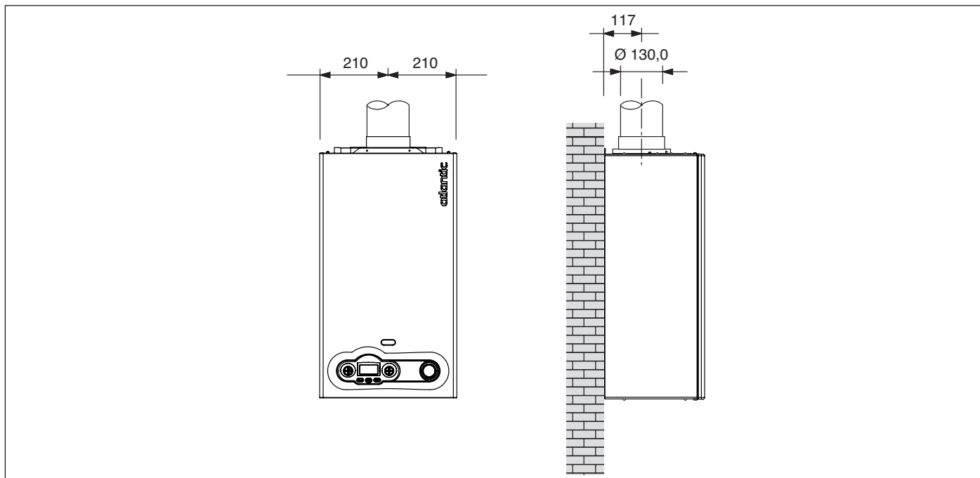
Fig. 6 données dimensionnelles pour le raccordement au conduit d'évacuation fumées
