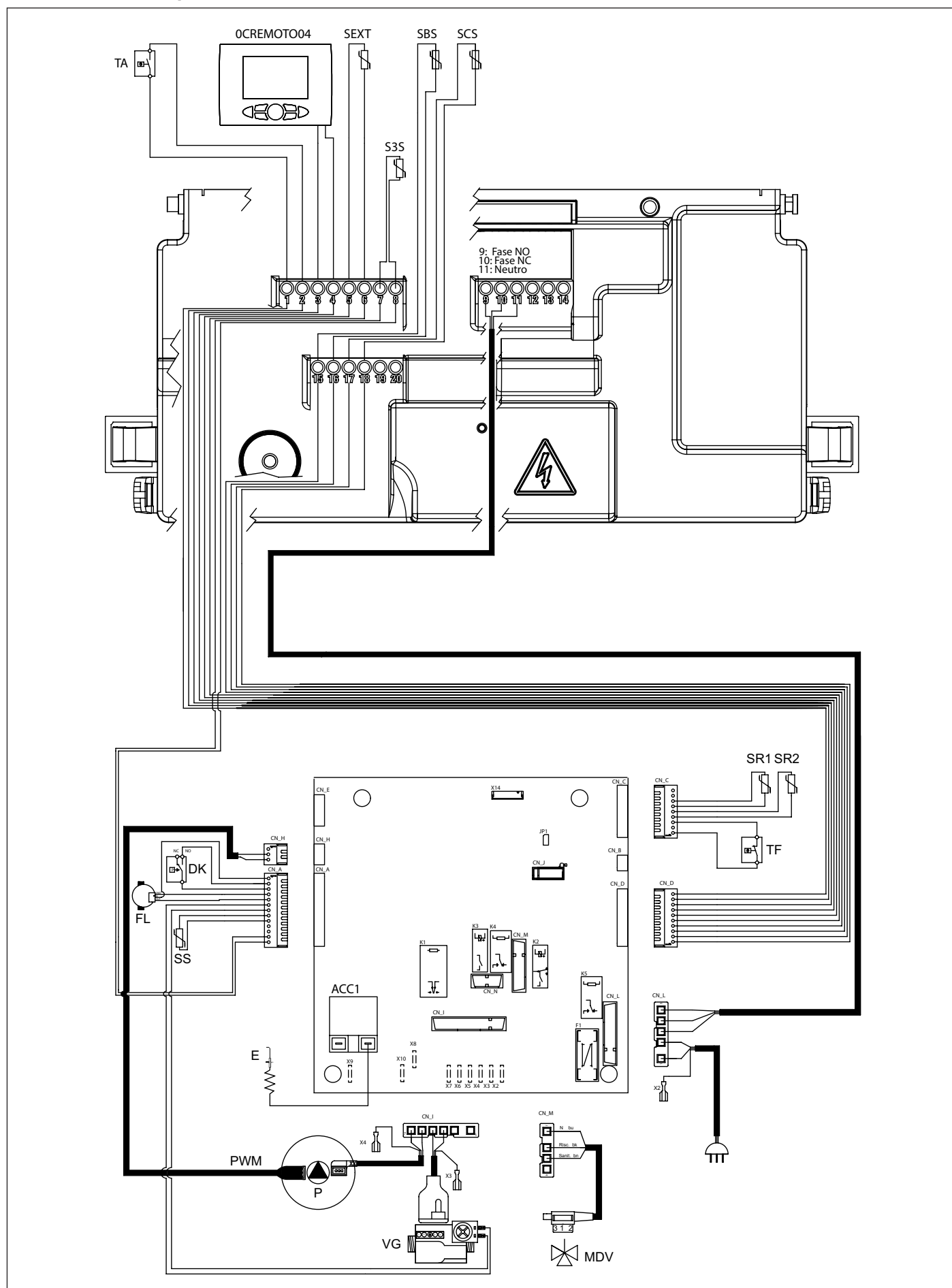
Fig. 11 Schéma électrique
