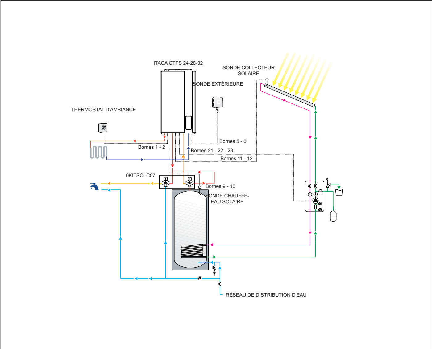
Fig. 12 Schéma de raccordement installation solaire à circulation forcée avec chaudière combinée
