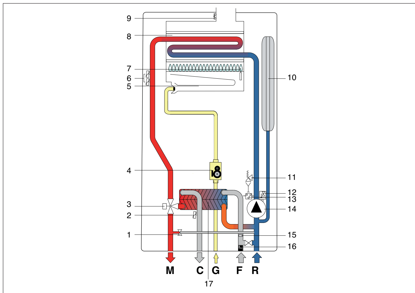
Fig. 3 Schéma hydraulique
