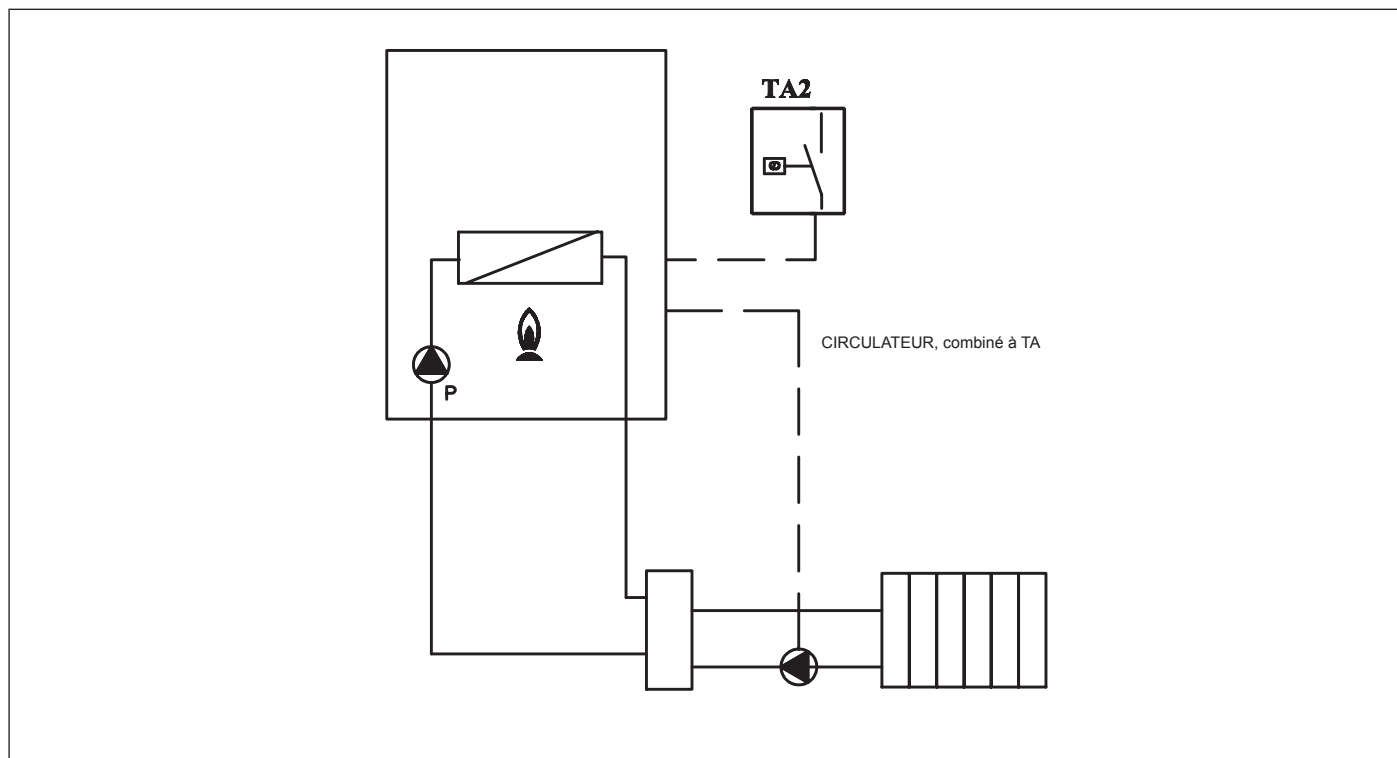
Fig. 16 Relais avec demande (P17=3)
