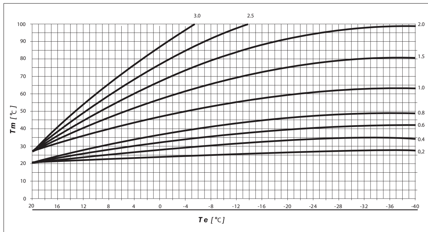
Fig. 8 Courbes de thermorégulation
