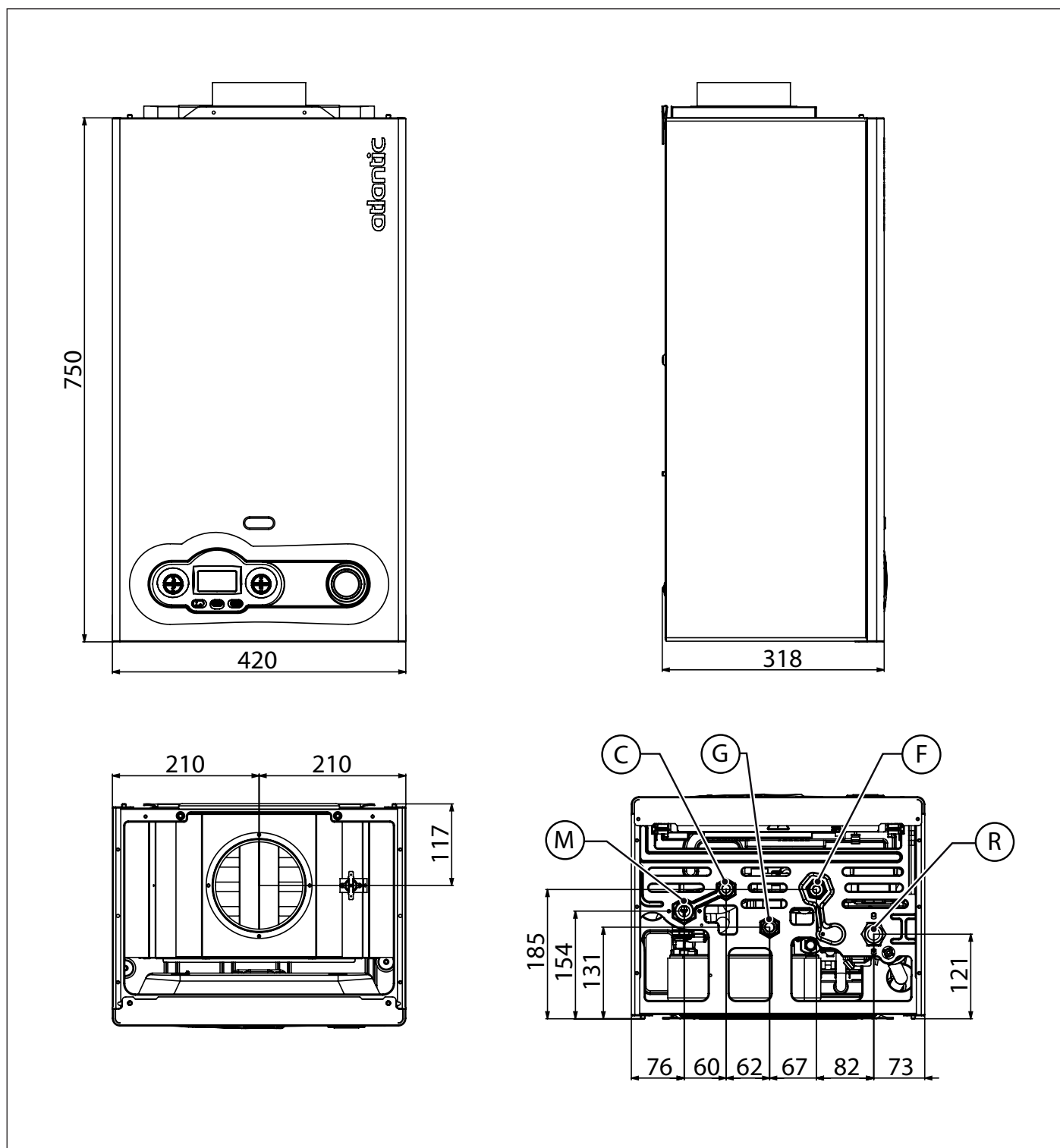
Fig. 2 Dimensions
