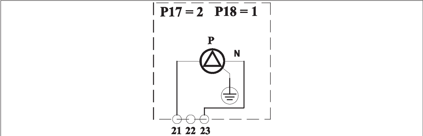
Fig. 13 Schéma de raccordement relais multifonction
