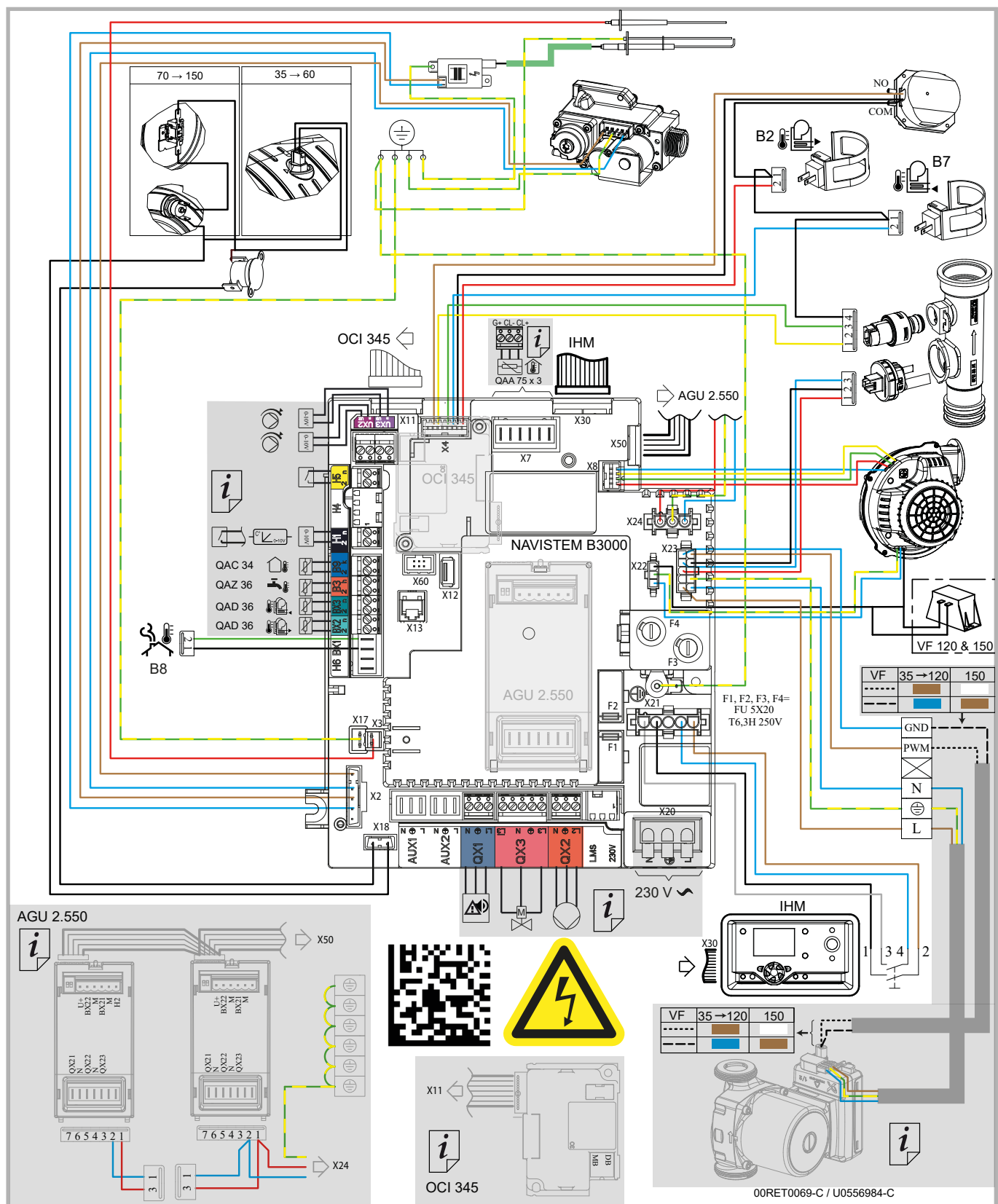
figure 23 - Schéma électrique
