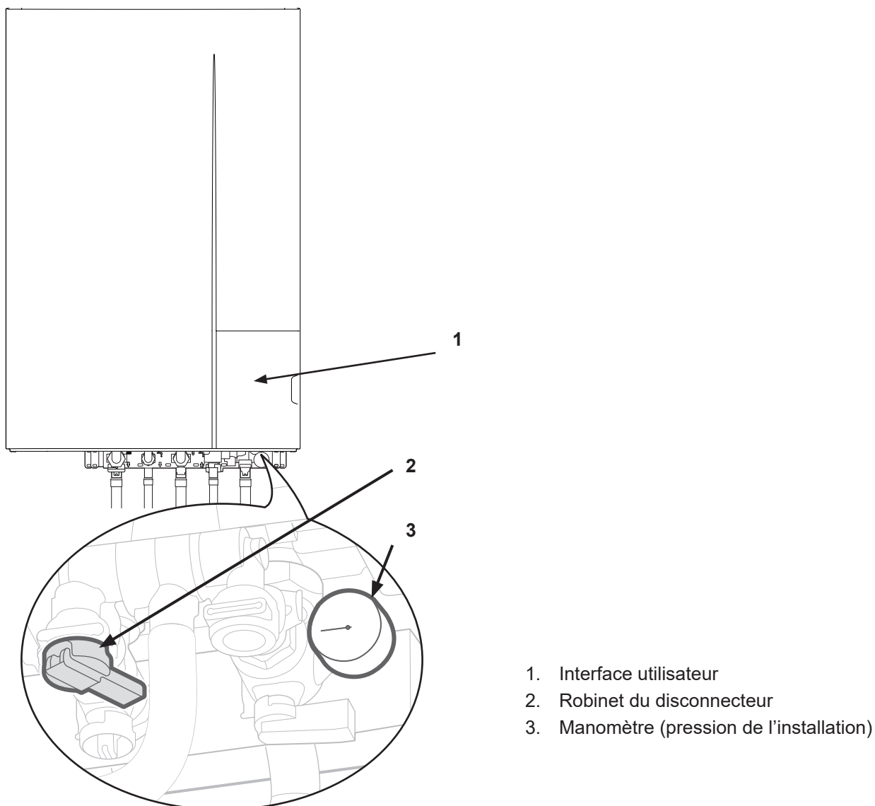
fig. 1 - Chaudière
