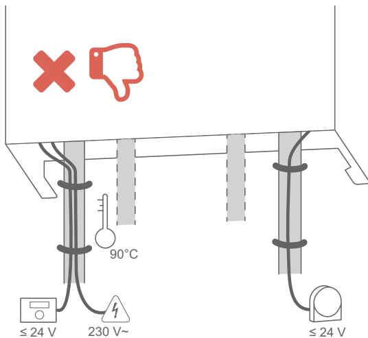
fig. 15 - Chemin de câbles
