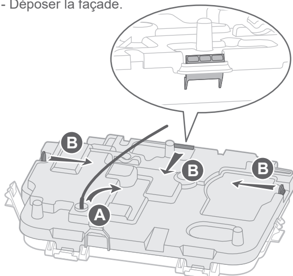
fig. 28 - Accès coffret électrique
