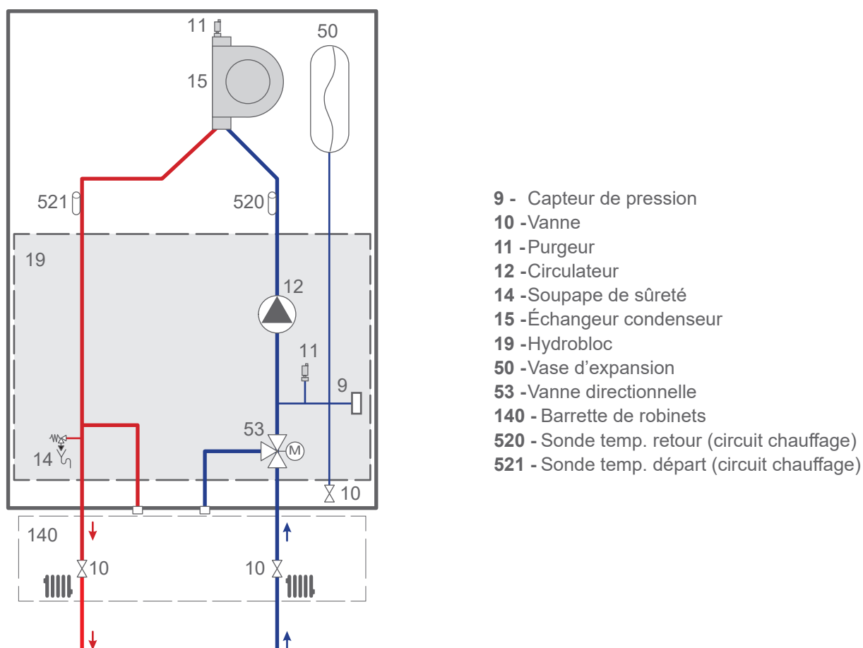
fig. 4 - Principe hydraulique
