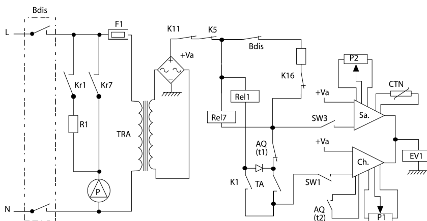
Schéma de câblage
