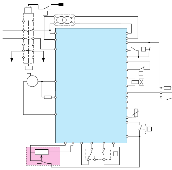
Schéma de câblage
