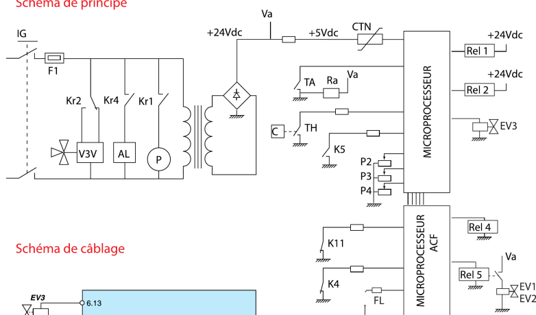
Schéma de principe
