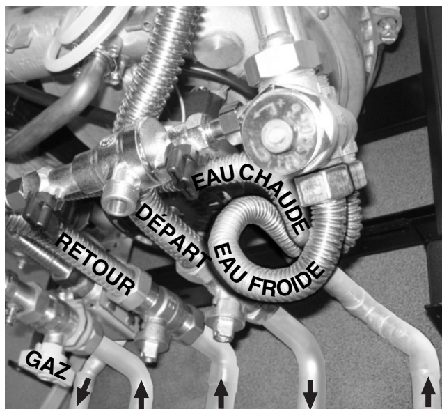
EAU CHAUDE 4 GAZ 1 RETOUR CHAUFFAGE 3 DEPART CHAUFFAGE 2 EAU FROIDE 5
