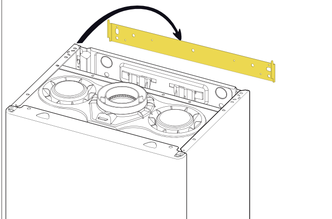
SCHÉMA 1 Installation Neuve sans cadre écarteur
