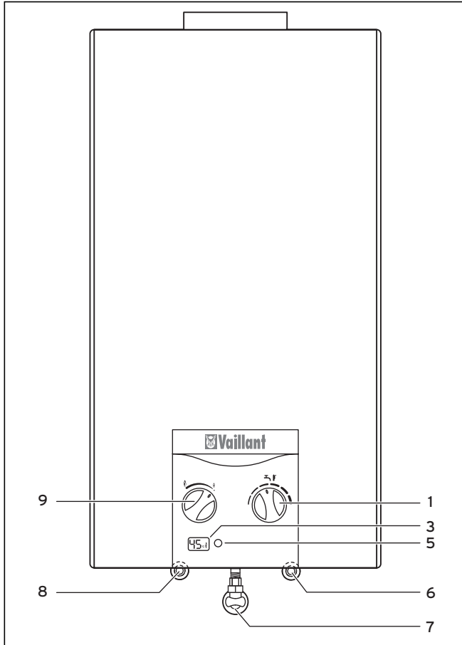
Fig. 4.1 Commandes atmoMAG
