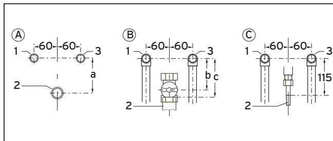
Fig. 4.1 Pré-installations murales
